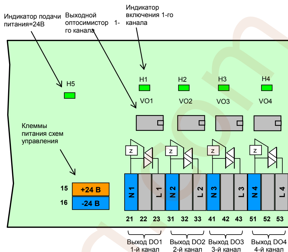
Рисунок Б.16 - Подключение дискретных нагрузок с помощью КБ3-28С-11
