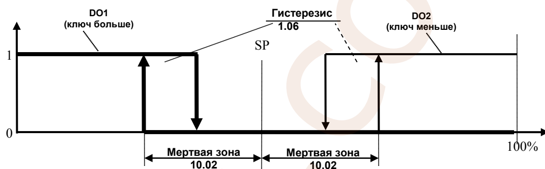
Рисунок В.8 - График работы дискретных выходов 3-х позиционного регулятора с использованием зоны нечувствительности (10.02)
