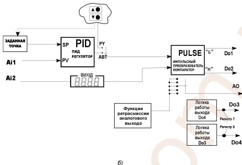
Рисунок 5.3 - Функциональная схема ПИД-импульсного блока регулирования МИК-21. а) – блок регулирования МИК-21 в случае если 10.13 ≠ 0003 (см. Приложение В), б) – блок регулирования МИК-21 в случае если 10.13 = 0003 (см. Приложение В),
