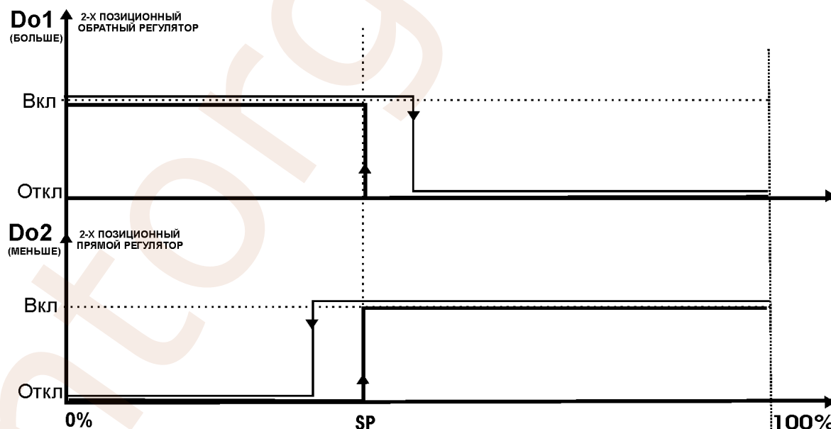
Рисунок В.9 - График работы 3-х позиционного регулятора с использованием гистерезиса без зоны нечувствительности 2-х позиционного прямого и обратного регулятора.
