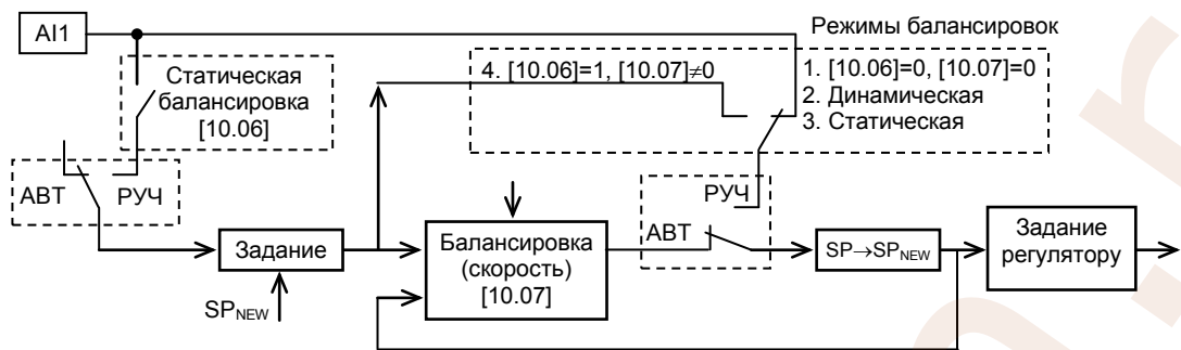
Рисунок 6.2. Функциональная схема балансировок регулятора МИК-21.
