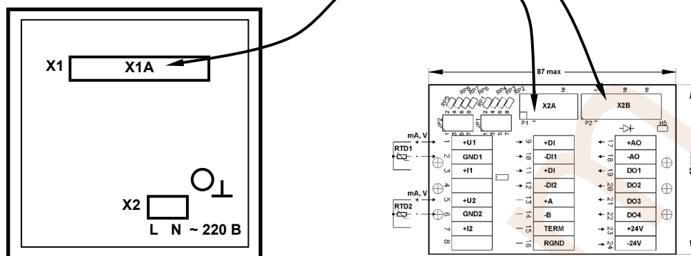
Рисунок Б.1 - Подключение клеммно-блочного соединителя KB3-25-11-0,75 к регулятору МИК-21-
