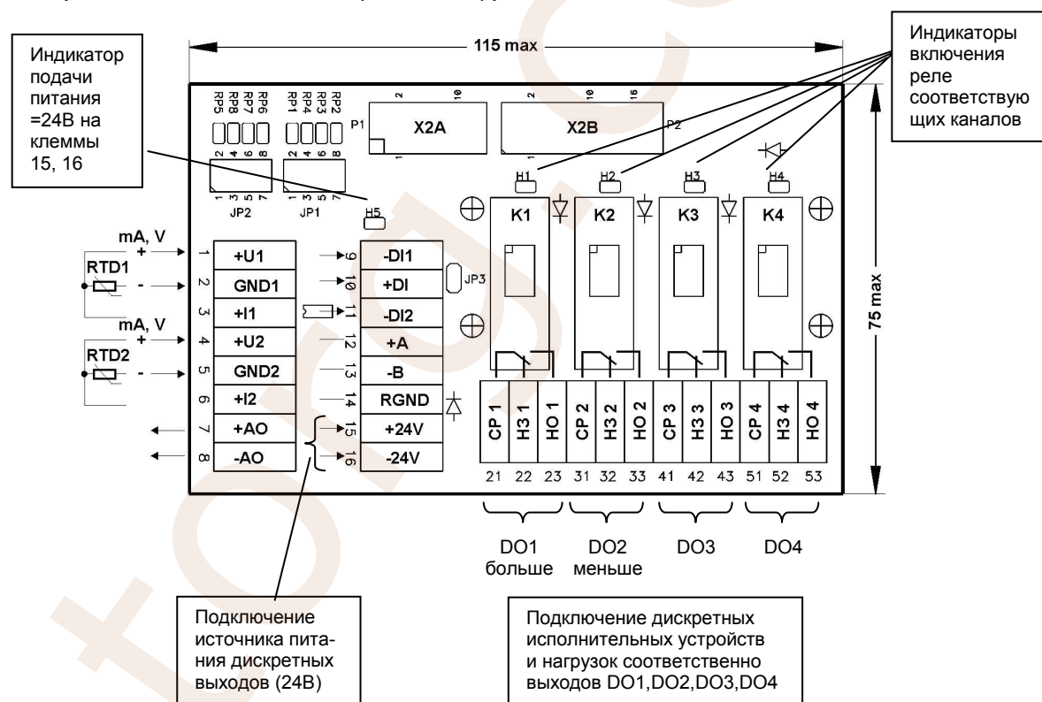
Рисунок Б.14 - Подключение дискретных нагрузок с помощью КБ3-28Р-11
