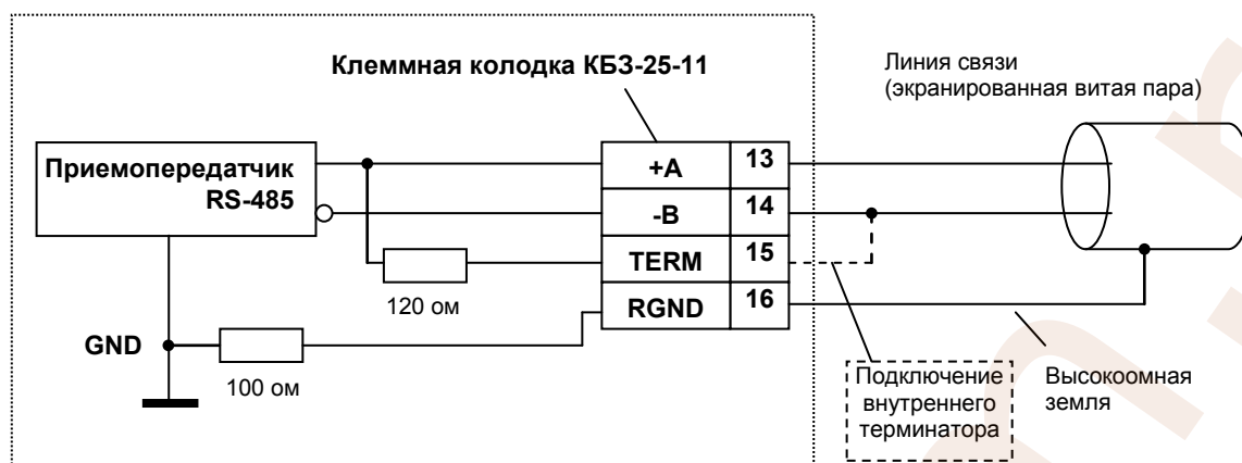
Рисунок Б.19 - Рекомендуемая схема подключения интерфейса RS-485 с помощью КБ3-25-11
