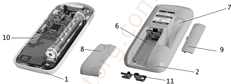
Рисунок 2 - Вид ззаду зі знятою нижньою накривкою
