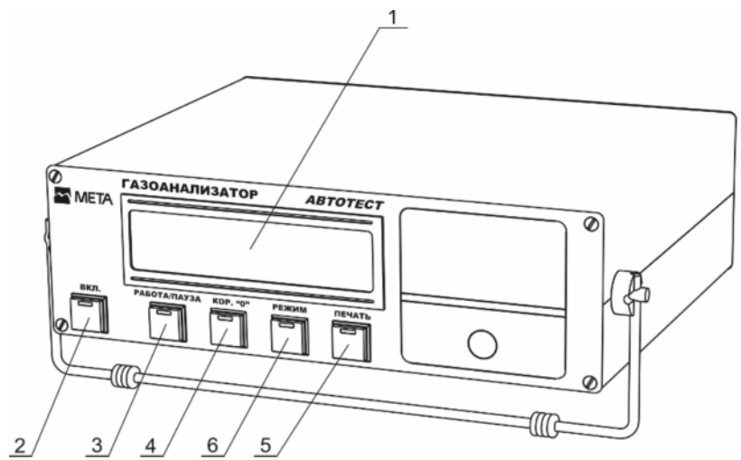
1-Индикатор; 2-Кнопка включения питания ВКЛ; 3-Кнопка РАБОТА/ПАУЗА; 4-Кнопка КОРР.0; 5-Кнопка ПЕЧАТЬ; 6-Кнопка РЕЖИМ
