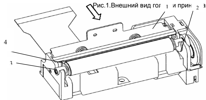
1 – Скоба-рычаг; 2 – Валик; 3 – Втулка; 4 – Термоэлемент
