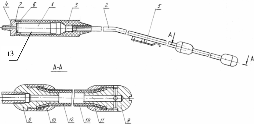
1-Фильтр; 2-Трубопровод; 3-Ручка; 4- Крышка; 5-Пружина; 6,7-Прокладка; 8-Штуцер; 9-Наконечник; 10,11- Втулка; 12-Трубка; 13-Колпачок; 14-Рукав
