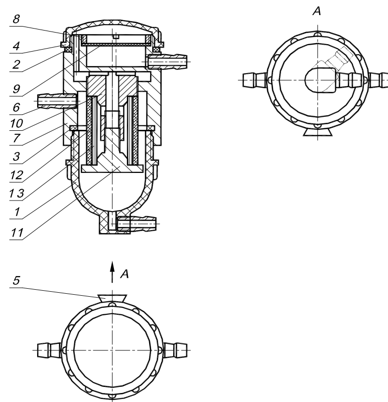
1-Колпачок; 2-Прокладка; 3-Прокладка; 4-Верхняя крышка; 5-Фиксатор; 6-Штуцер подачи газа; 7- Корпус; 8-Гайка; 9-Диск бумажного фильтра; 10-Оправа; 11-Фиксатор; 12-Фильтр 5 мкм; 13 Объемный фильтр
