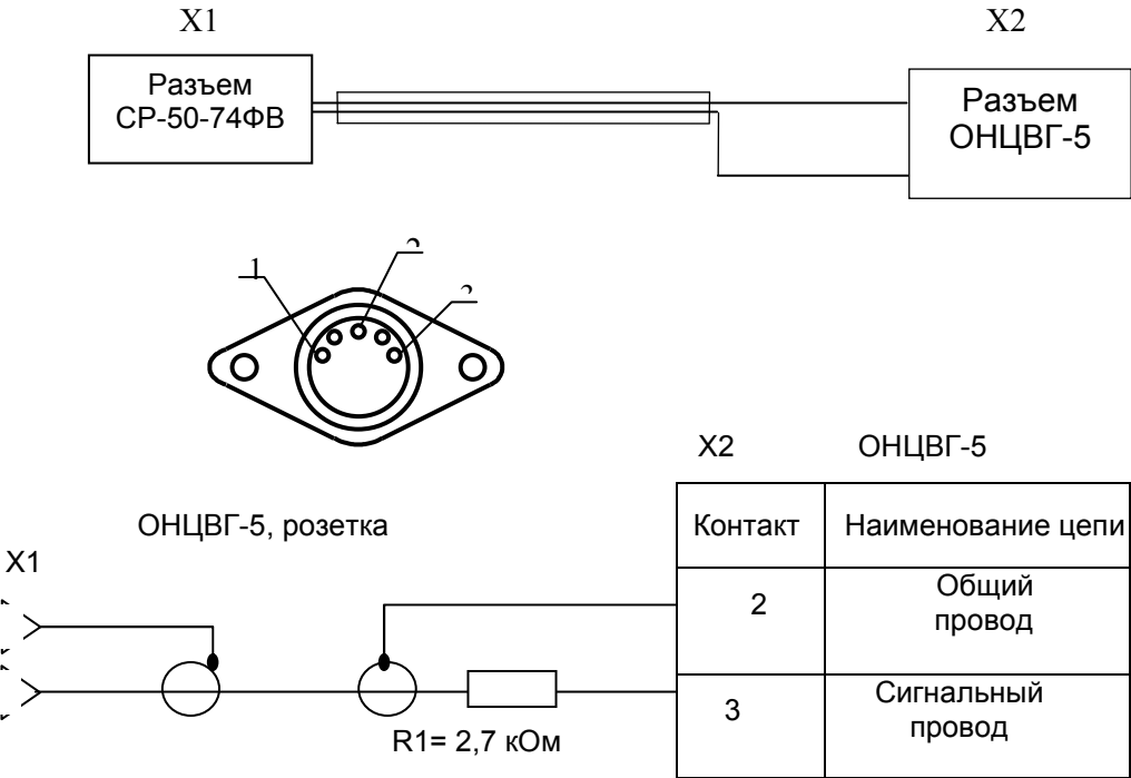
Рис.4. Конструкция и схема кабеля для поверки канала тахометра
