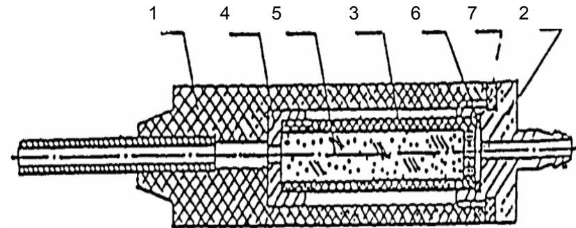
1-Рукоятка; 2-Штуцер; 3-Патрон; 4-Крышка патрона; 5-Фильтрующий агент (стекловолокно); 6,7-Прокладка Рисунок 2 - Пробозаборник
