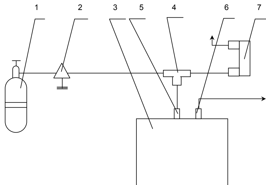
1 - Баллон ПГС 2 - Вентиль тонкой регулировки 3 - Прибор 4 - Тройник 5 - Штуцер "Вход" 6 - Штуцер "Выход" 7 - Расходомер
