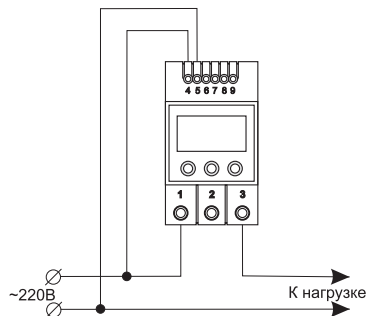
Схема подключения
