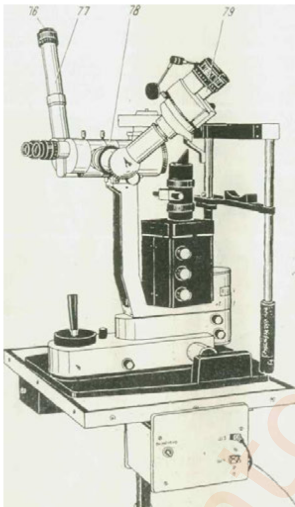
Общий вид щелевой лампы с комплектом оптических насадок
