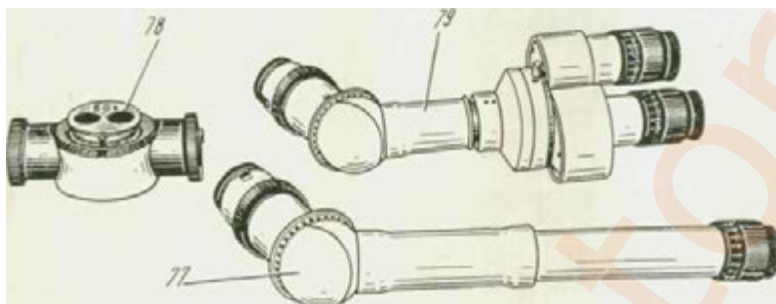
77 — монокулярная трубка; 78 — оптический делитель; 79 — бинокулярная трубка
