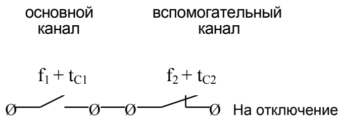
Рисунок В.3 – Соединение контактов реле частоты УРЧ в режиме БССЧ
