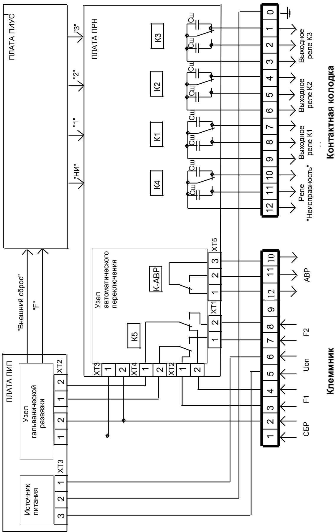
Рисунок А.3 – Подключение внешних цепей реле УРЧ-3М-С-02 через контактную колодку и клеммник к внутренним элементам реле
