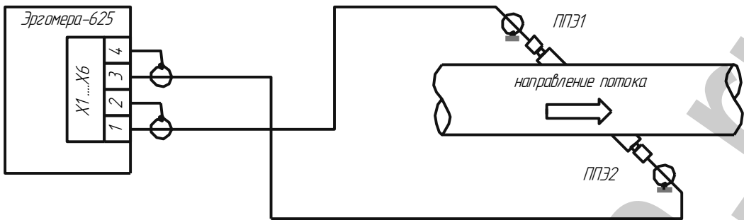
Подключение датчиков УЗ-расходомеров 1..6 к клеммам счётчика X1..X6
