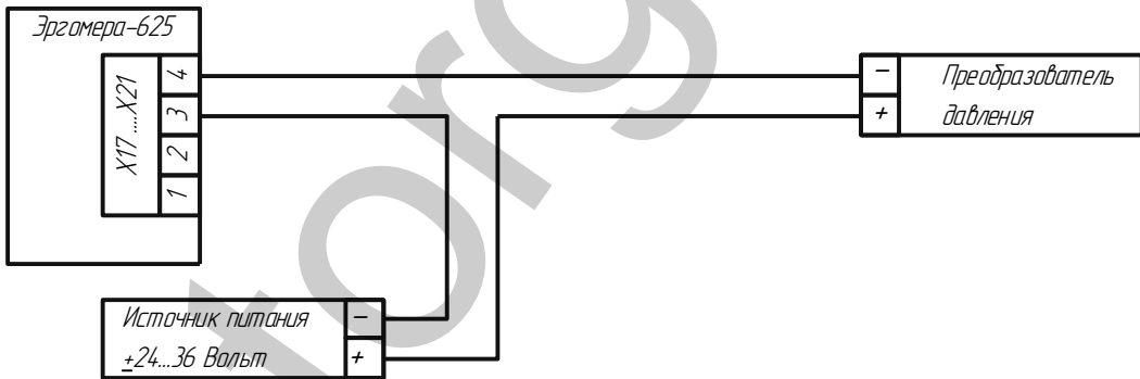
Подключение преобразователей давления с токовым выходом к клеммам счётчика X17..X21
