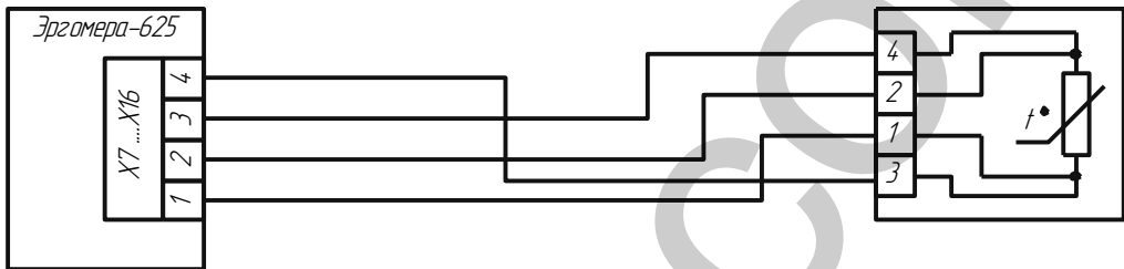
Подключение термопреобразователей сопротивления 1..10 к клеммам счётчика X7..X16
