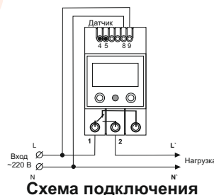
Схема подключения
