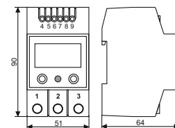
Габаритные размеры
