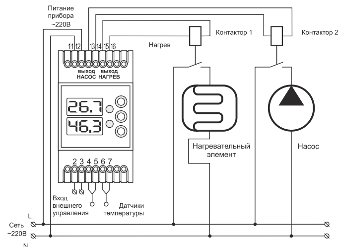
Назначение выводов
