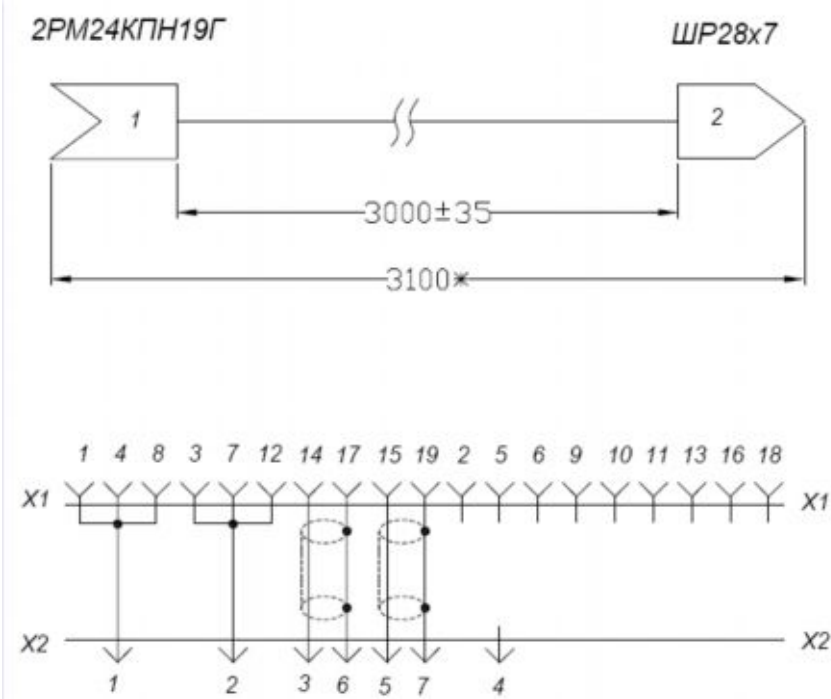
Рисунок Б.4. Схема кабеля питания и измерительных сигналов.
