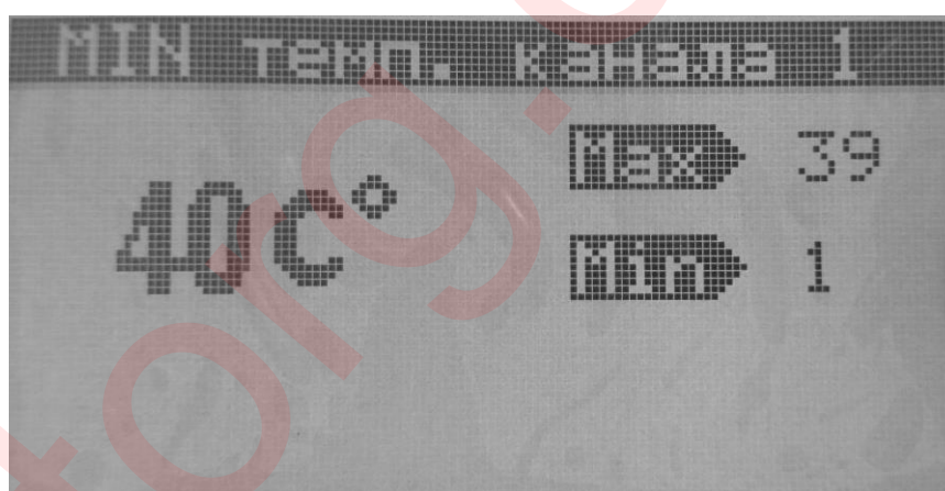
Рисунок 22 – Окно изменение параметра MIN температура
