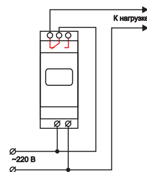
Схема подключения реле
