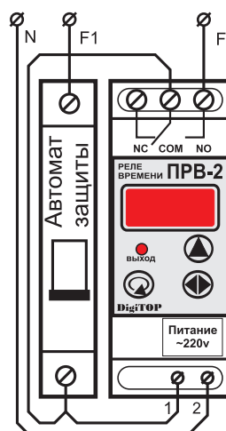
Монтажная схема подключения реле
