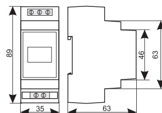
Габаритные размеры
