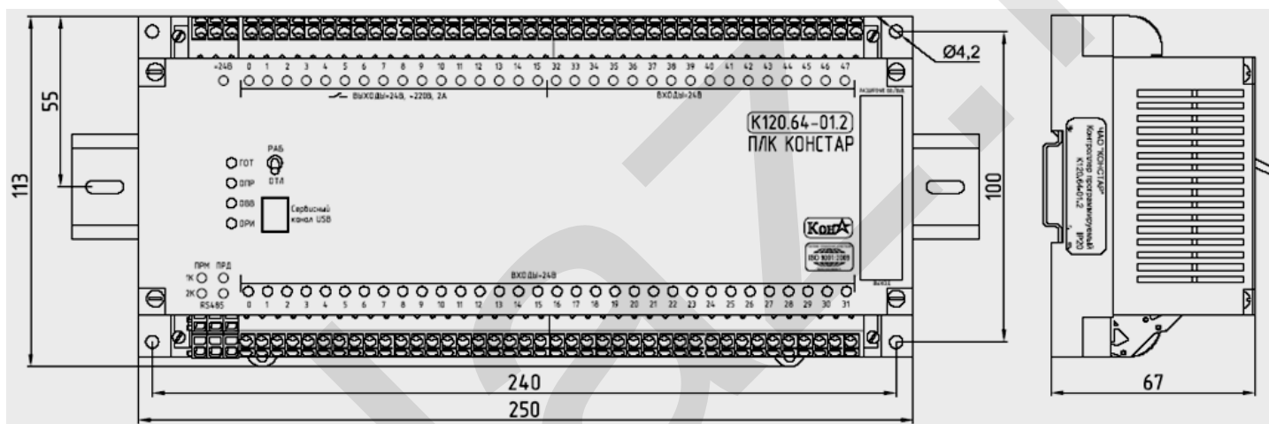
Рисунок 2.4.3. Габаритные и установочные размеры блока K120.64-01.2
