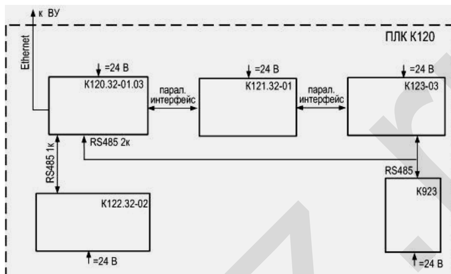
Рисунок 5.2.1 Структурная схема ПЛК K120
