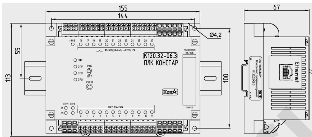
Рисунок 2.4.2. Габаритные и установочные размеры блока K120.32-06.3
