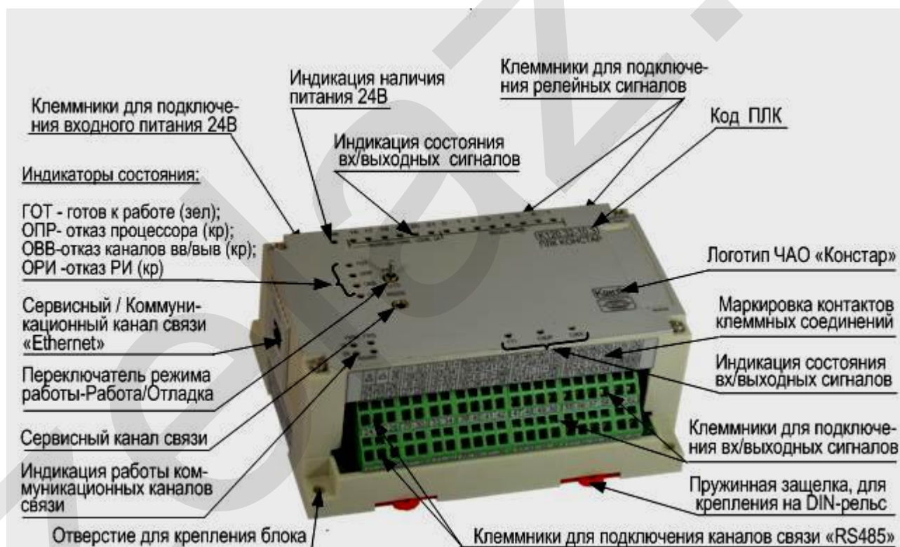
Рисунок 2.4.1. Внешний вид базового блока ПЛК К120 с пружинными клеммниками
