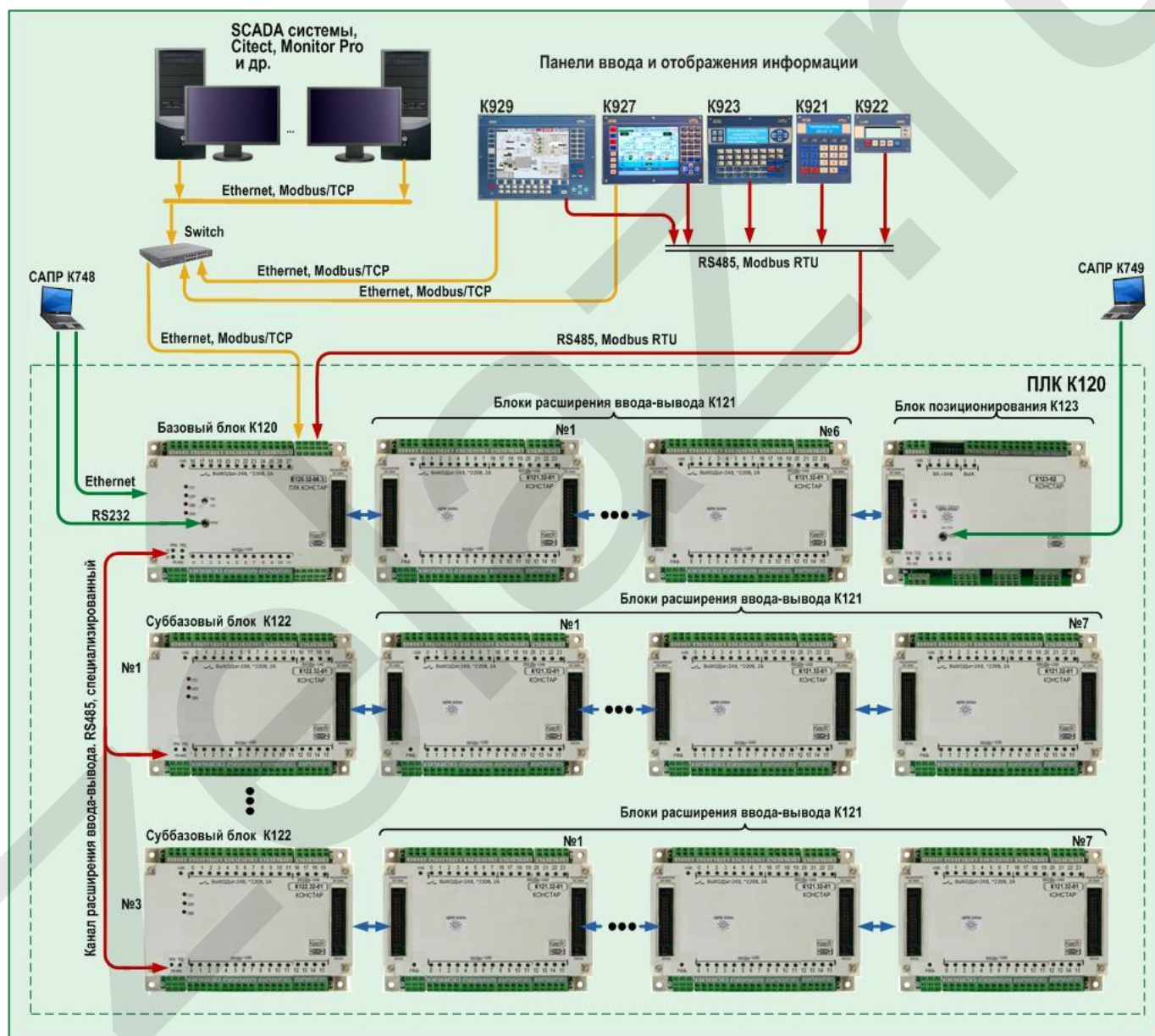
Рисунок 2.3.1. Одна из возможных структурных схем подключения ПЛК K120
