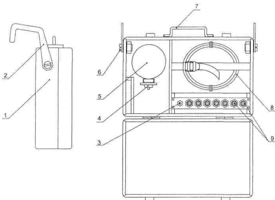
1-Ящик, 2-Скоба, 3-Ниппель, 4-Штуцер манометра, 5-Манометр, 6-Винт, 7-Ручка, 8-Шланг, 9-Штуцер
