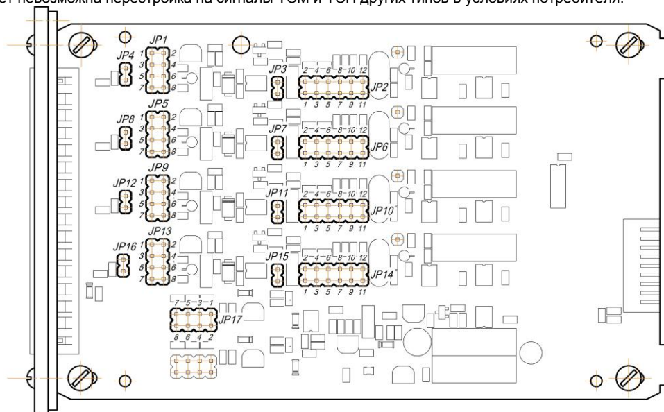
Рисунок 8.5.1 – Положение перемычек на плате аналоговых входов контроллеров МИК-50-16 и МИК-50-17
