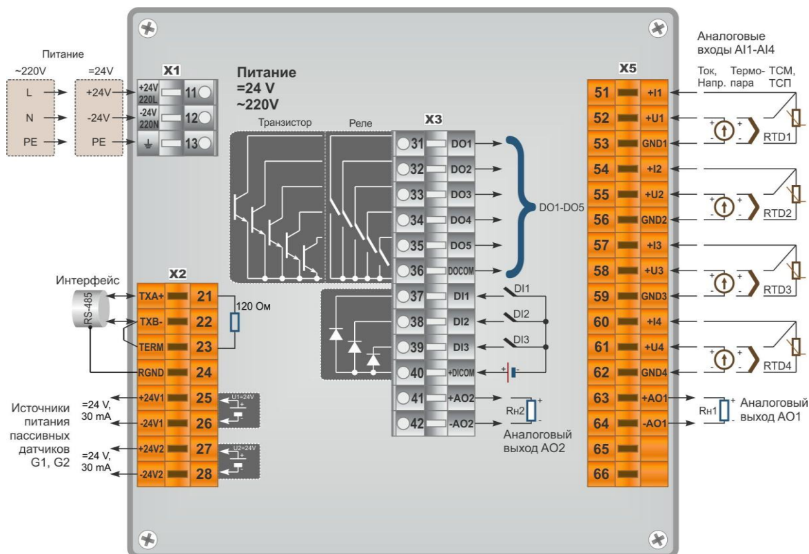
Рисунок 8.1 - Нумерация клемм и сигналы контроллера МИК-50-16
