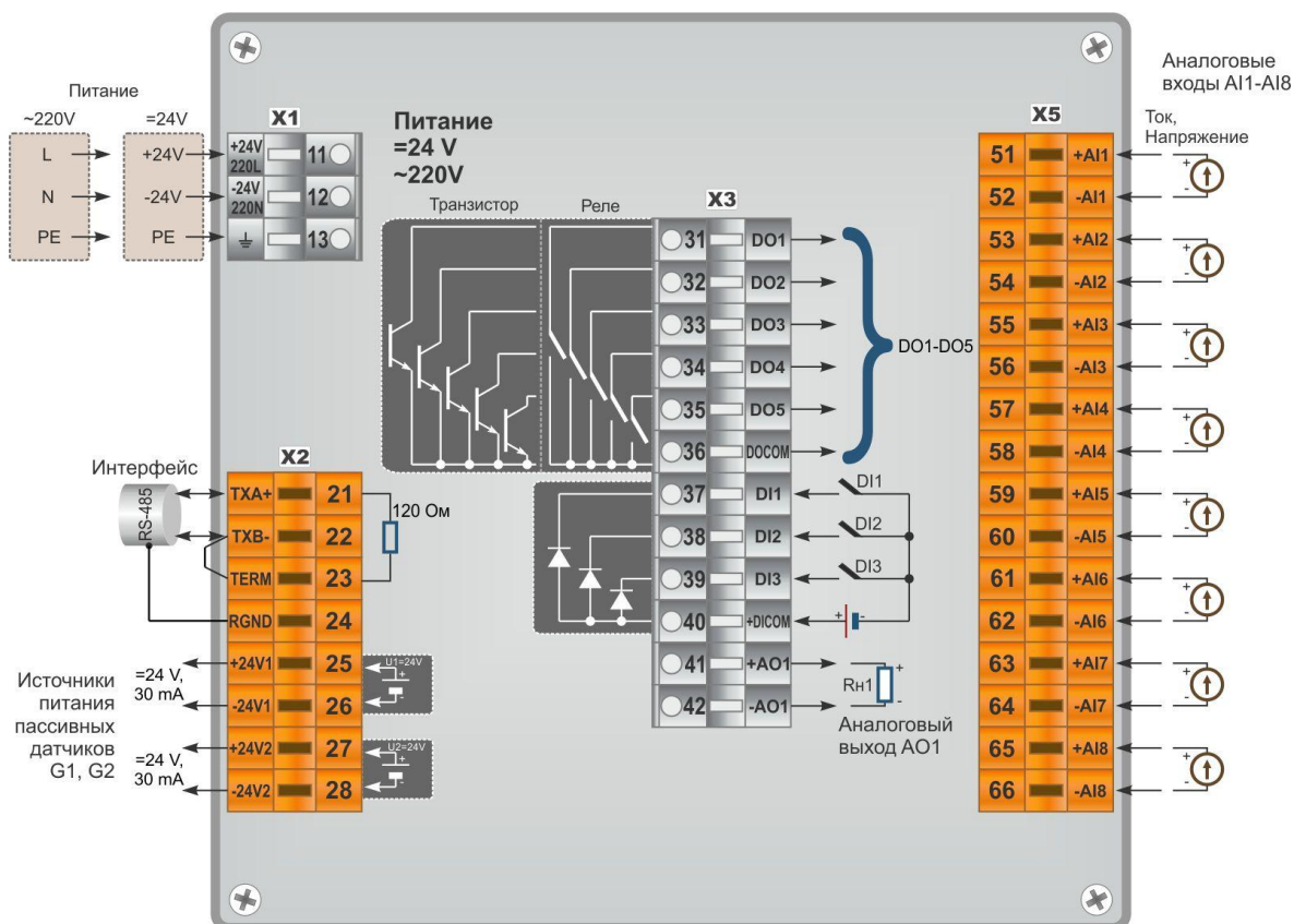
Рисунок 8.3 - Нумерация клемм и сигналы контроллера МИК-50-26
