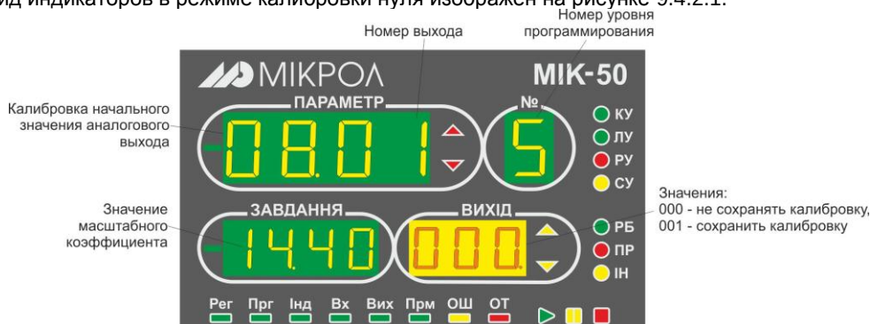
Рисунок 9.4.2.1 - Внешний вид индикаторов при калибровке начального значения аналогового выхода
