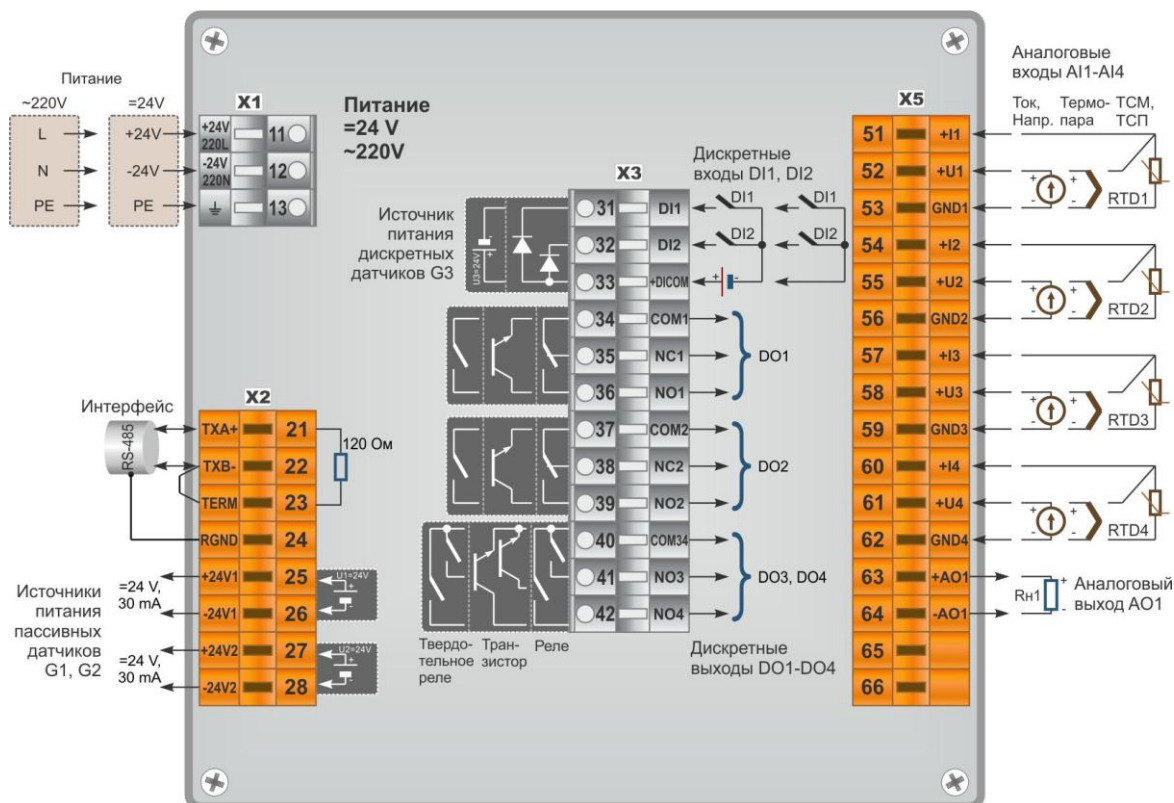
Рисунок 8.2 - Нумерация клемм и сигналы контроллера МИК-50-17
