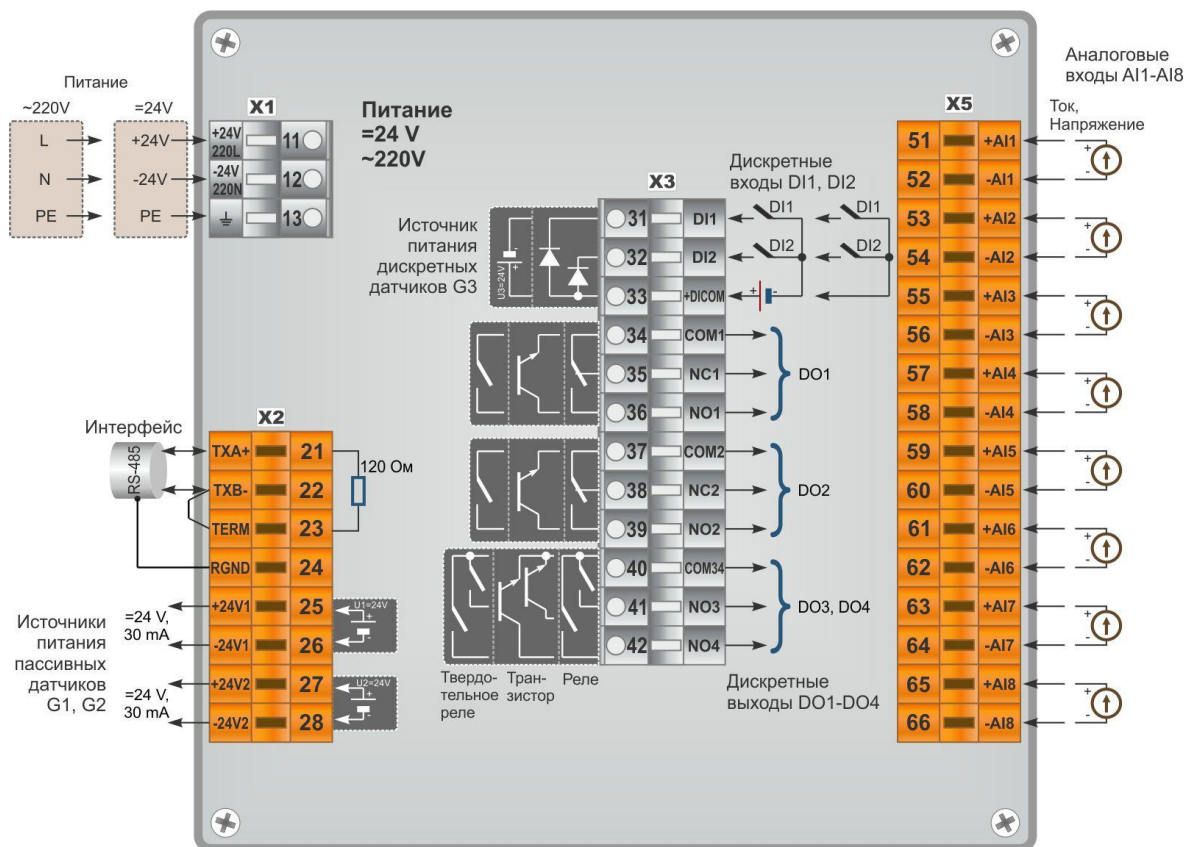
Рисунок 8.4 - Нумерация клемм и сигналы контроллера МИК-50-27
