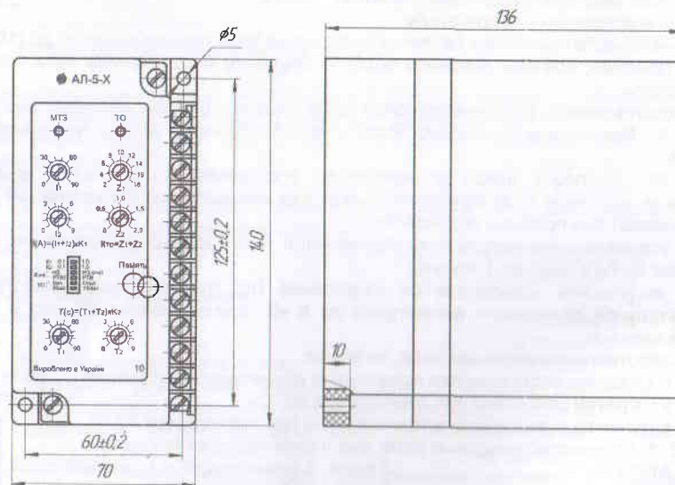
Рисунок 1 - Габаритные и установочные размеры реле АЛ-3-ОВ и АЛ-5Х
