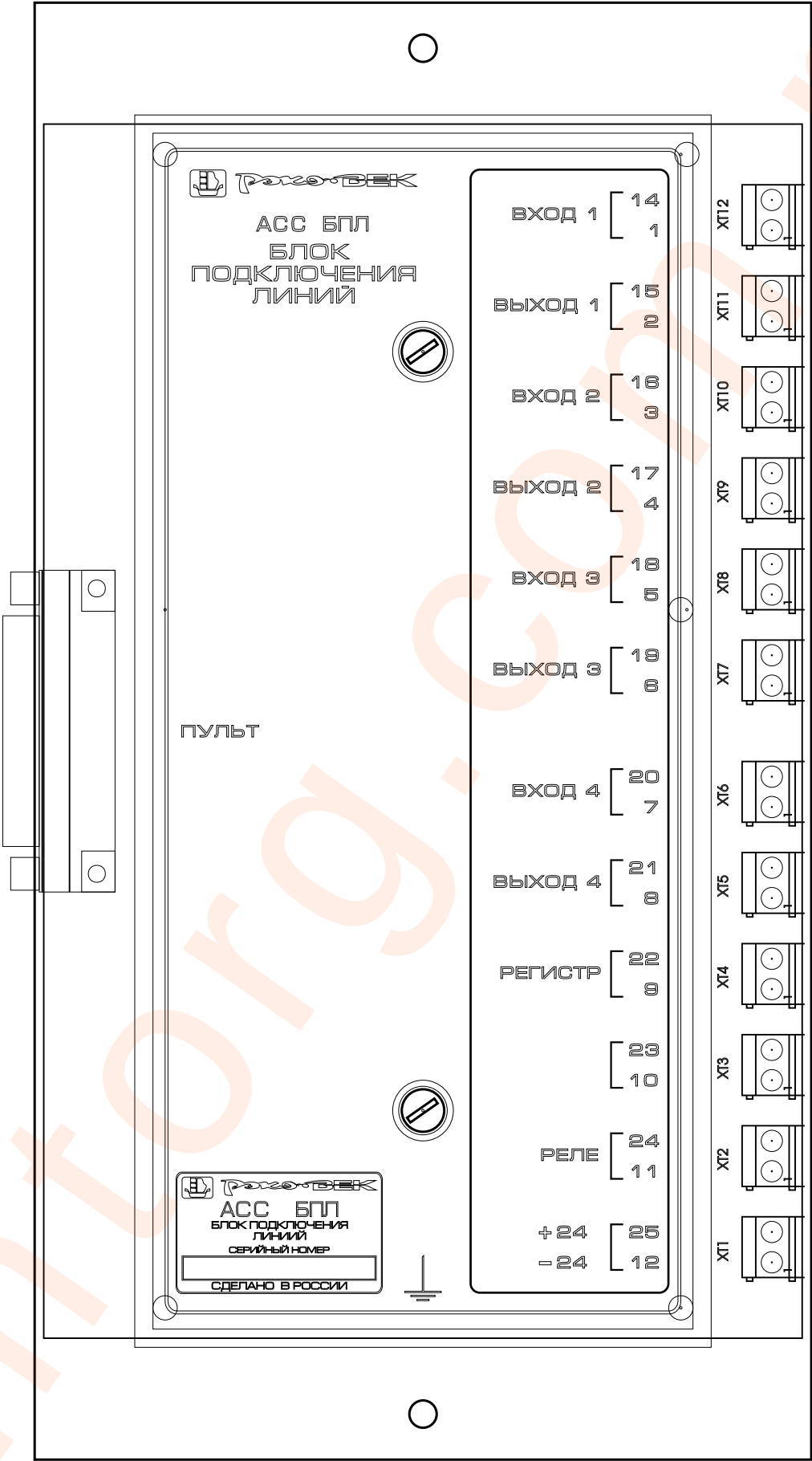
Внешний вид блока подключения линий БПЛ
