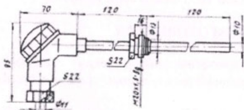
Термопреобразователь сопротивления ТСМ-1088
