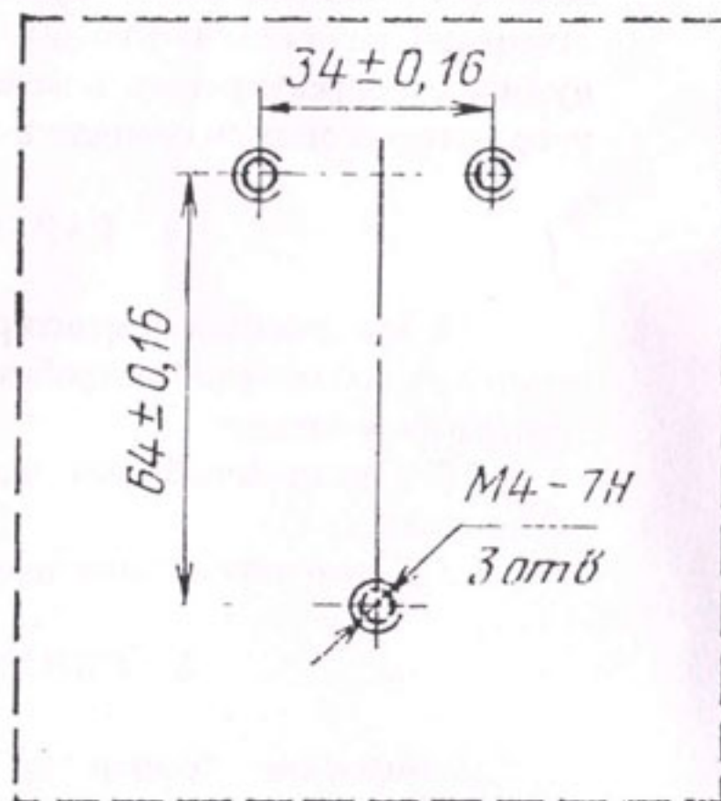
Разметка под крепление
