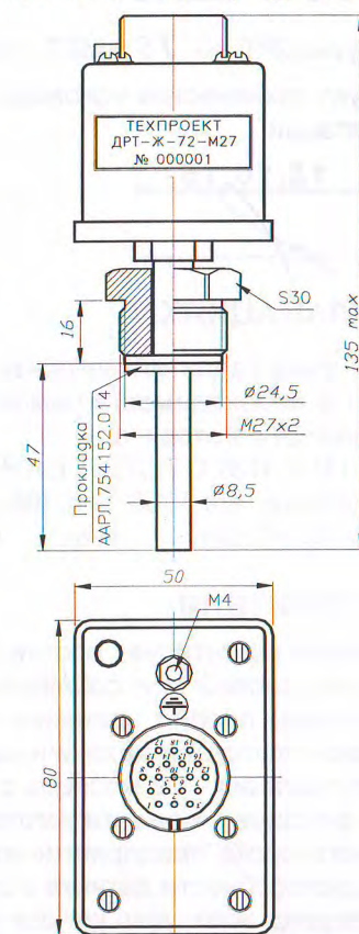
Рисунок 1 – Габаритные размеры ДРТ-Ж-...-М27.
