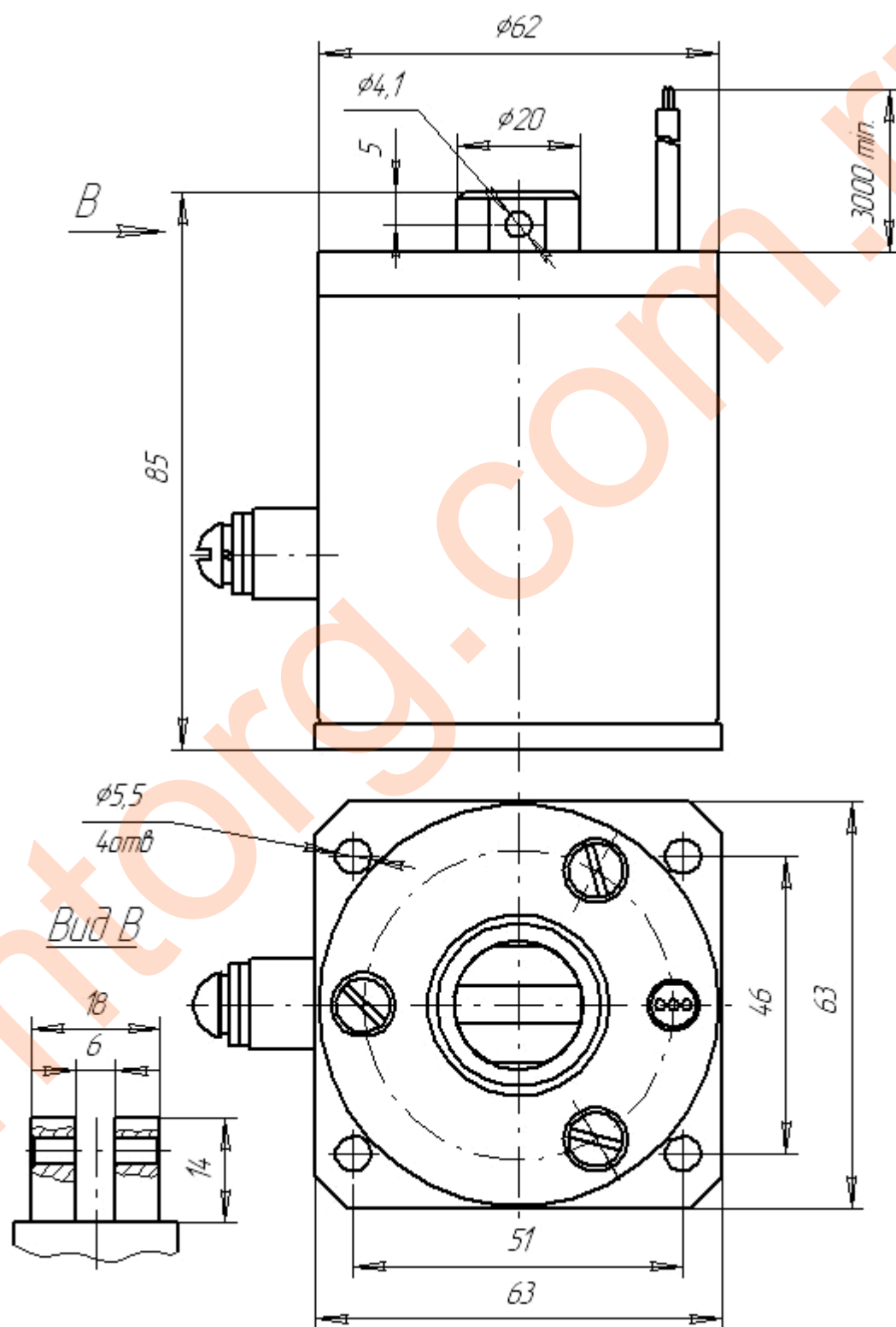
Электромагнит ЭМД 2 В3
