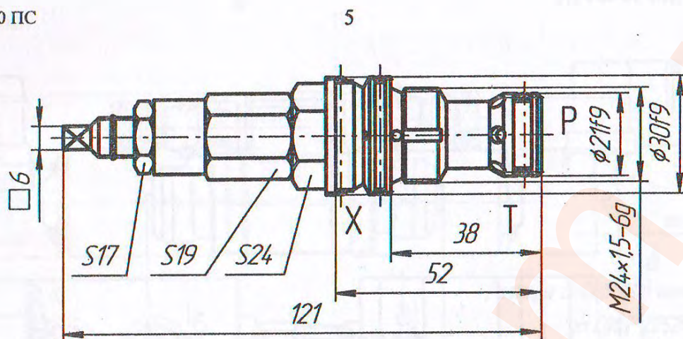
Рисунок 1.4 - Габаритные и присоединительные размеры клапана предохранительного типа КПР 10/X ВВ3 - X1
