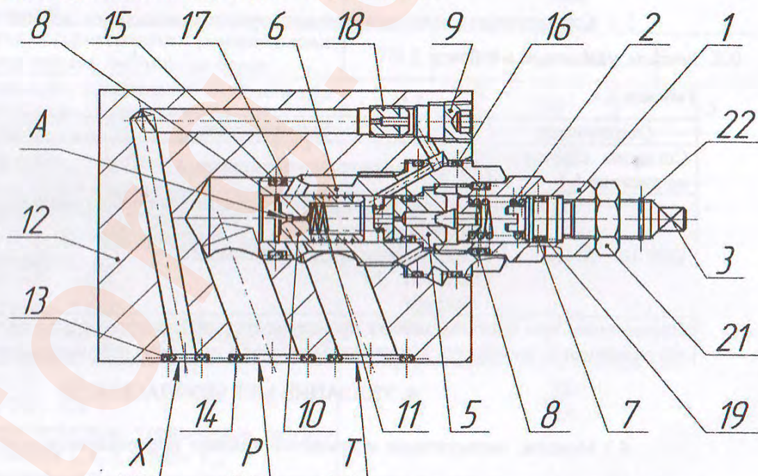
Рисунок 5.1 Конструкция клапана предохранительного типа КПр 10
