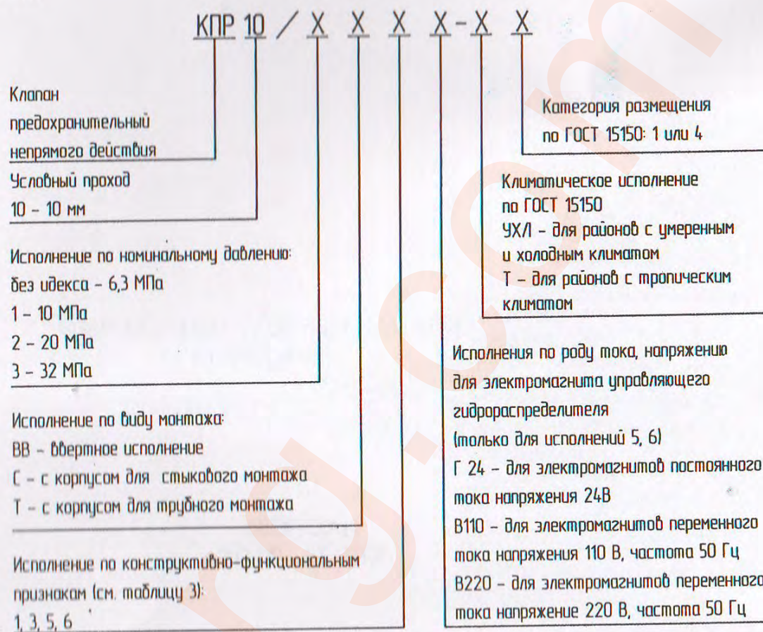
Рисунок 1.1 Условное обозначение гидроклапанов предохранительных
