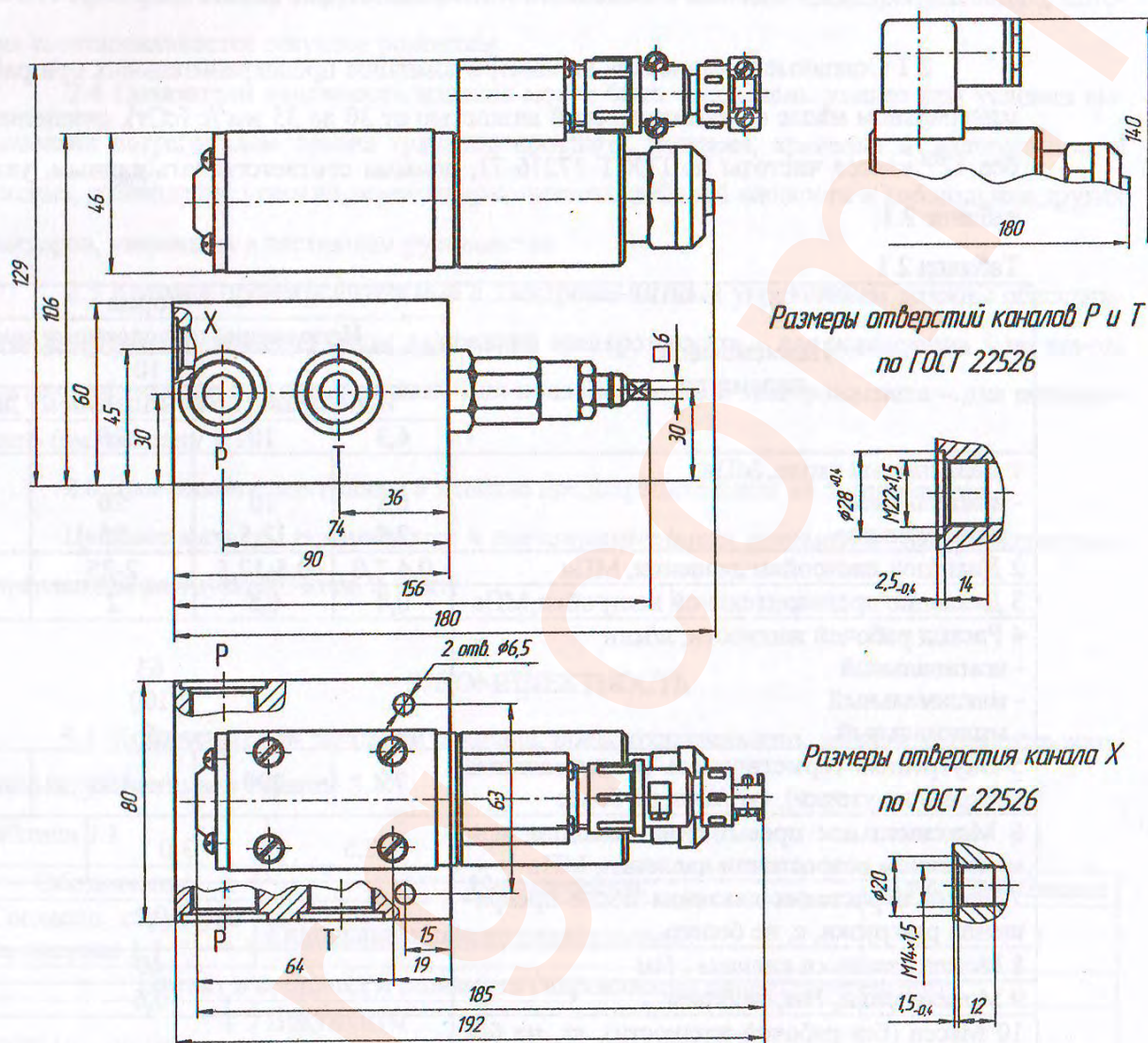
Рисунок 1.4 - Габаритные и присоединительные размеры клапана предохранительного типа КПР 10/X TXX – XX
