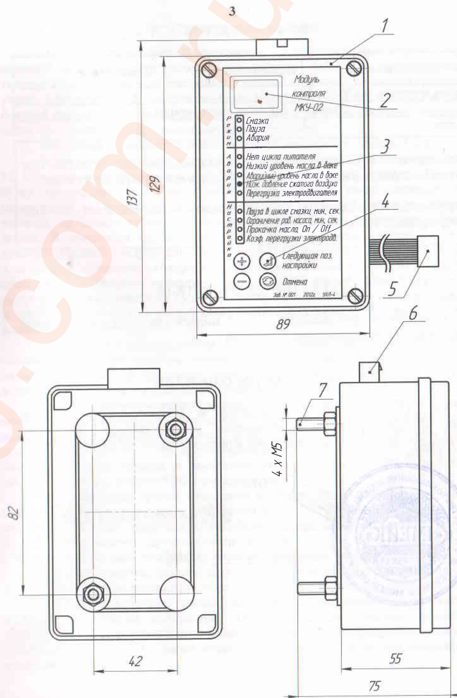
Рисунок 1 - Модуль контроля МКУ-02
