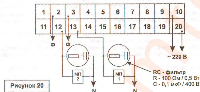
СХЕМА ПОДКЛЮЧЕНИЯ
