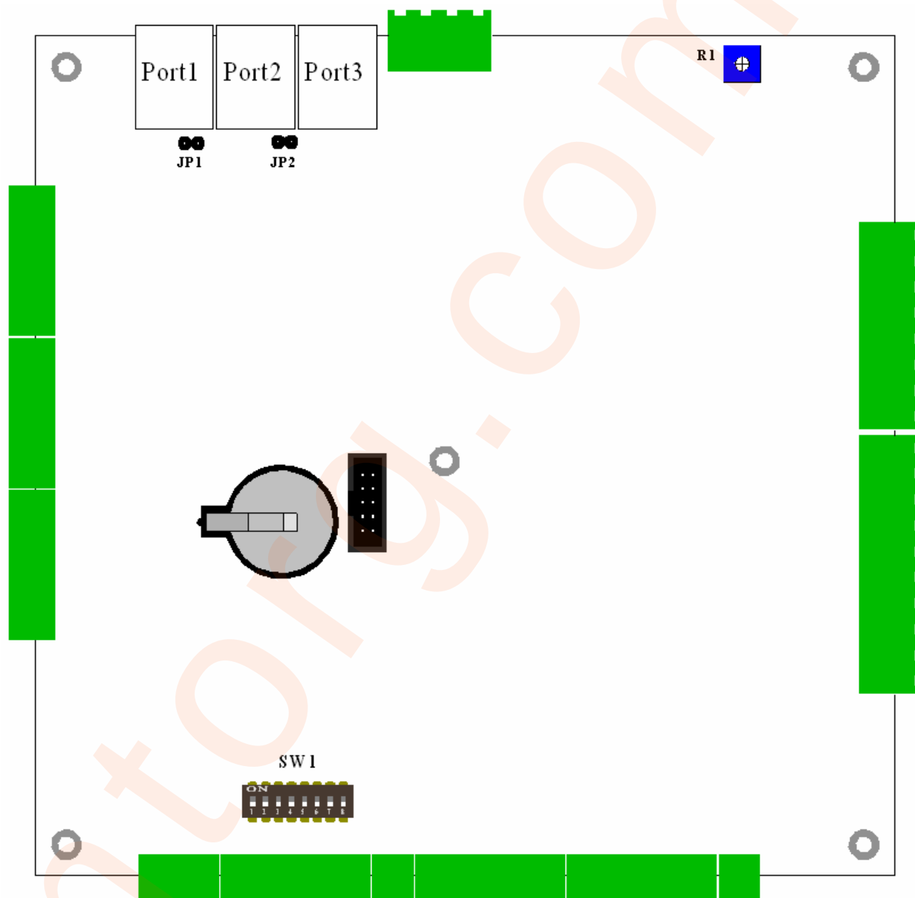
4.9. Выбор интерфейса для порта 1 и порта 2 производится автоматически без использования джамперов. Интерфейс порта 3 только RS232. Порт 3 предназначен для подключение GSM-модема пр-ва «ЭЛАС».
