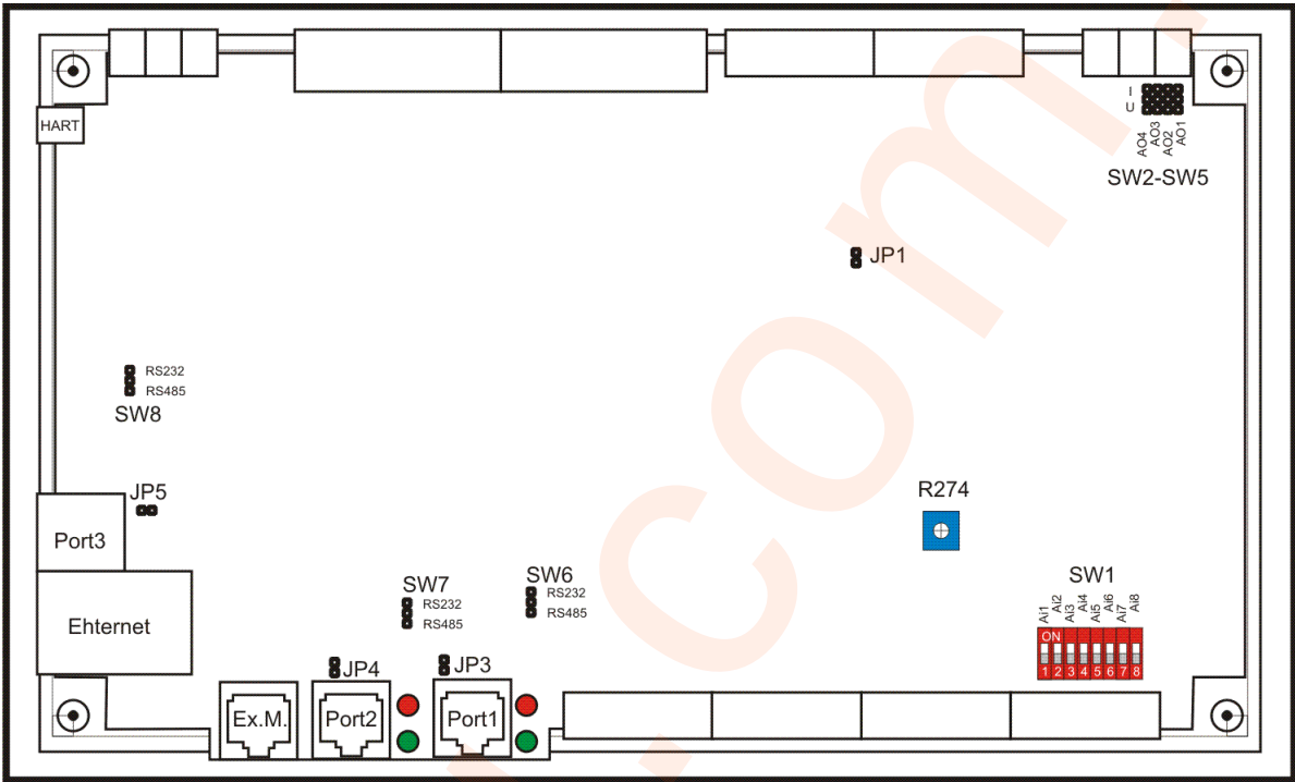
Рис.2. Расположение настроечных элементов на печатной плате.
