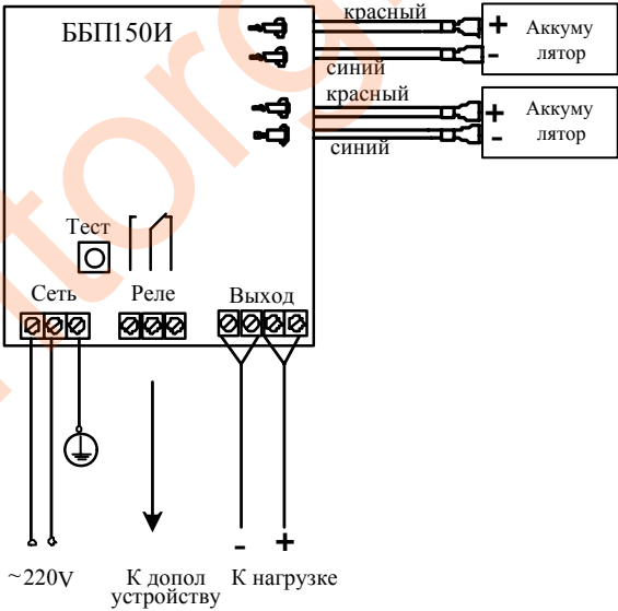
Приложение Б. Схема внешних соединений
