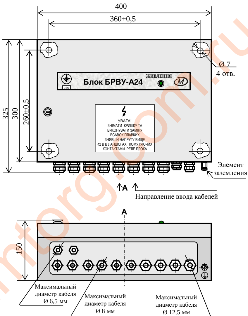
Рисунок 1 - Блок БРВУ-А24
