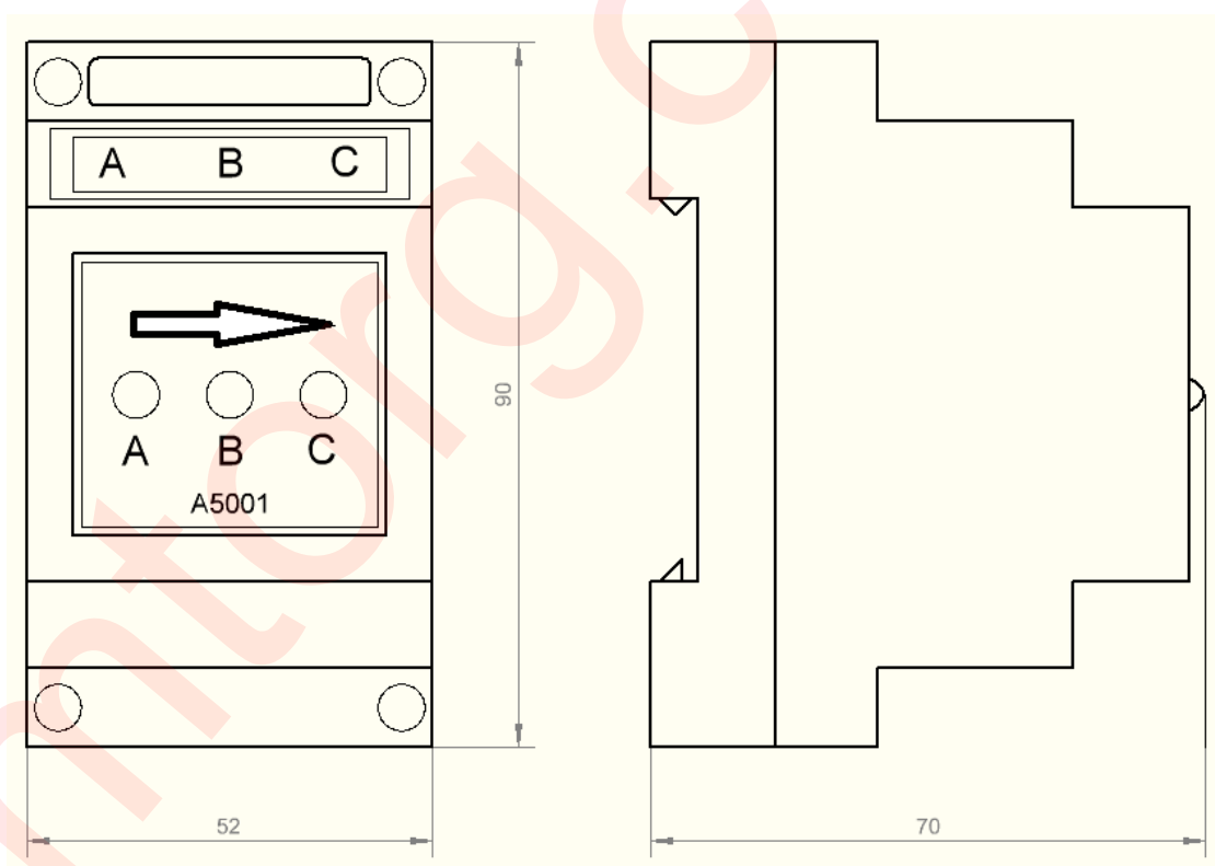
Рис. 6.1 - Внешний вид и габаритные размеры фазоуказателя
