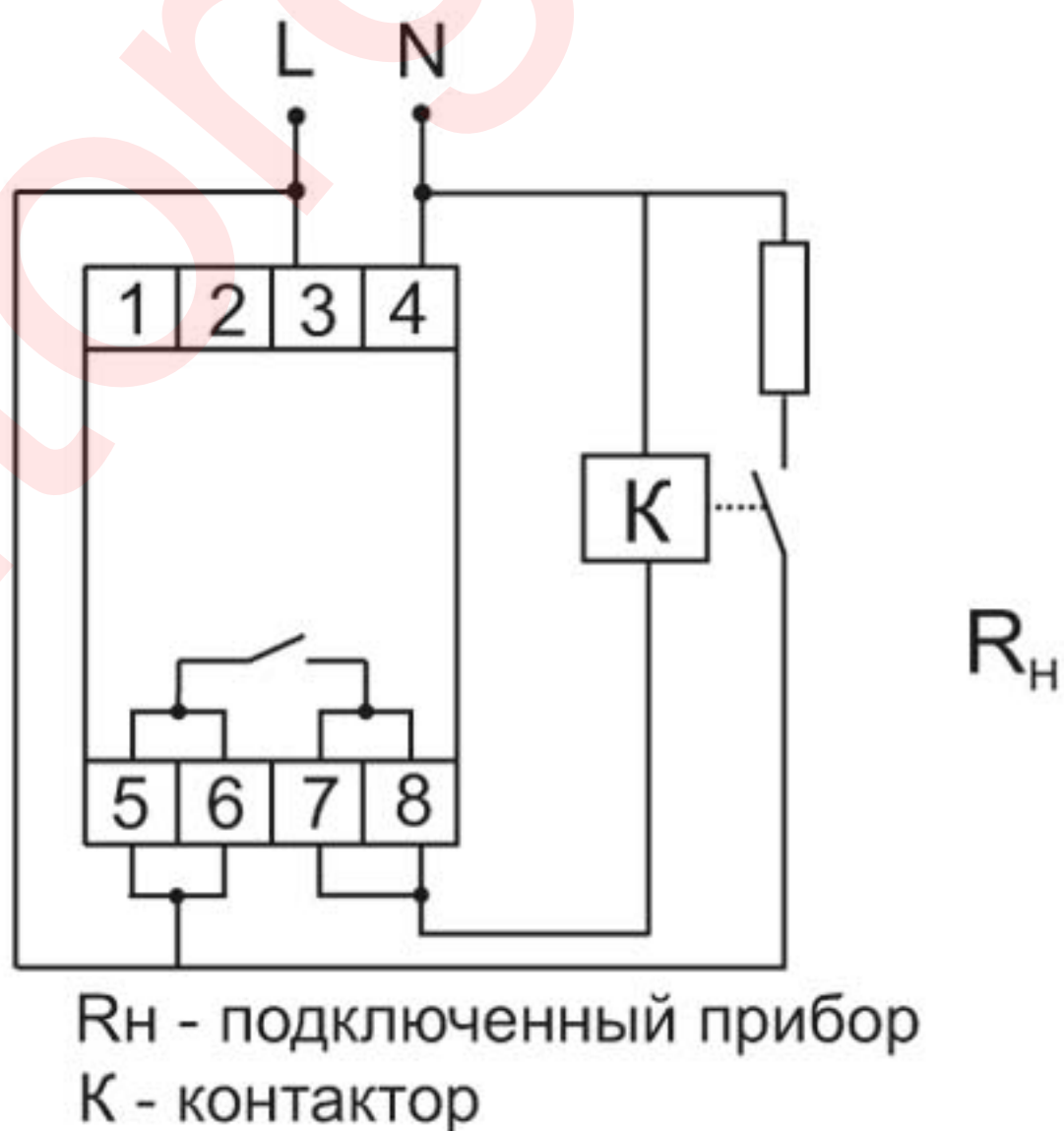
Рис.2 С применением контактора при потребляемом токе нагрузки более 30 А AC1
