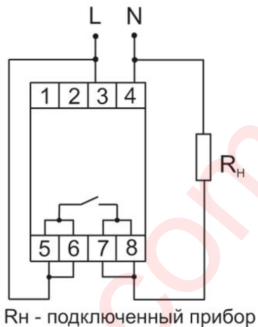
Рис. 1 При используемой нагрузке до 30 А AC1
