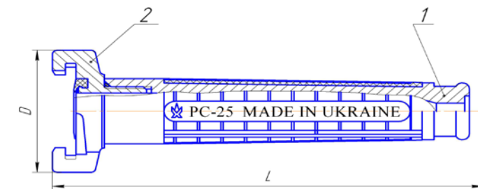
1- корпус; 2 – головка соединительная
