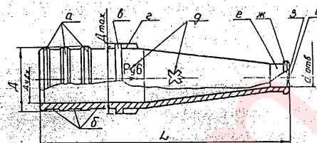
Ствол ручной для внутренних пожарных кранов
