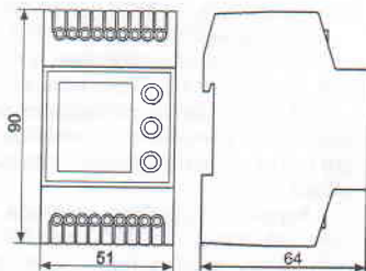
Габаритные размеры
