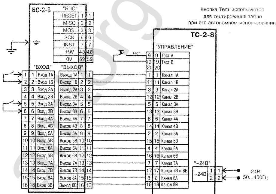
Рисунок 2 – Схема подключения табло совместно с блоком BS-2-8
