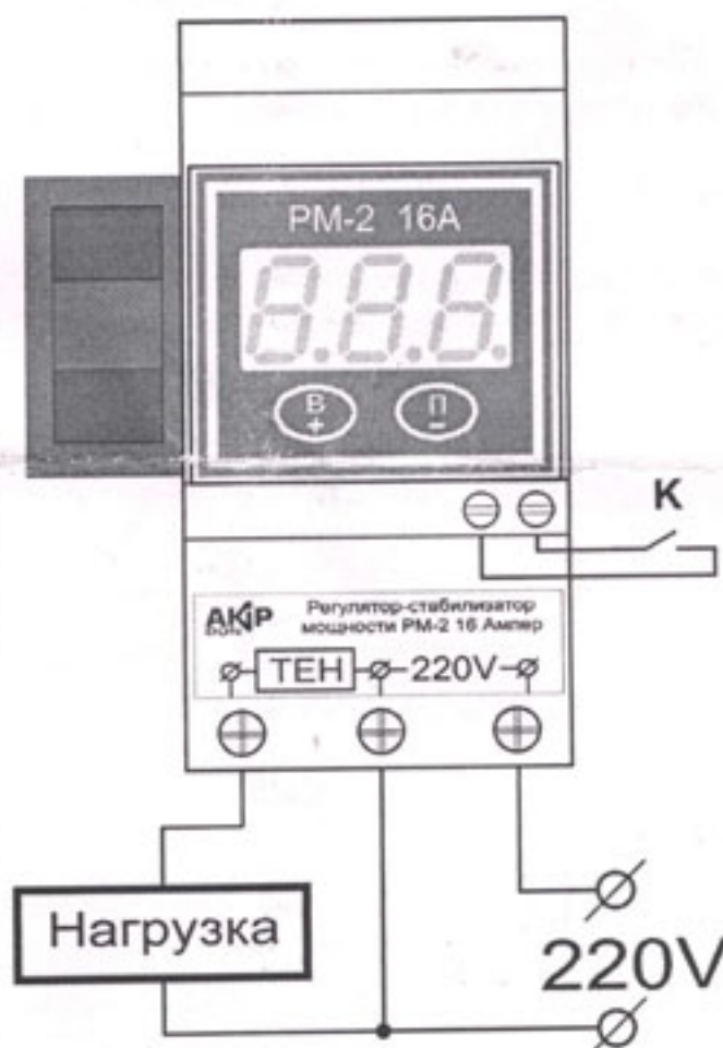
Рис. 1. Схема монтажа прибора.
