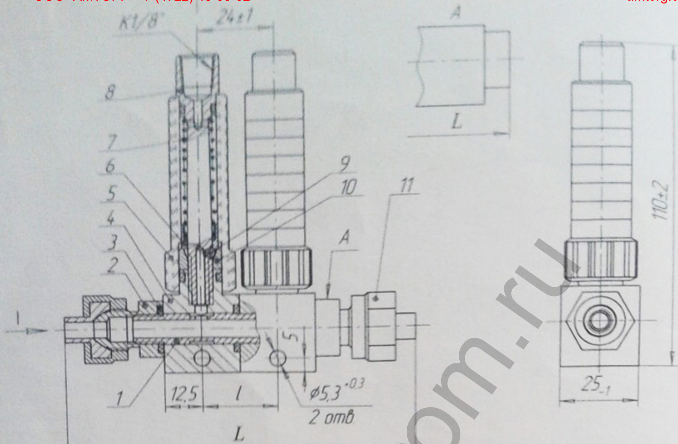
1-шпилька; 2-штуцер; 3-кольцо; 4-корпус; 5-трубка; 6-поплавок; 7-пружина; 8-стержень; 9-шарик; 10-гайка; 11-соединения для сообщения с трубопроводом \varnothing 8 \times 1 ; А – для блоков с одним подводом; I-подвод; II-отвод
