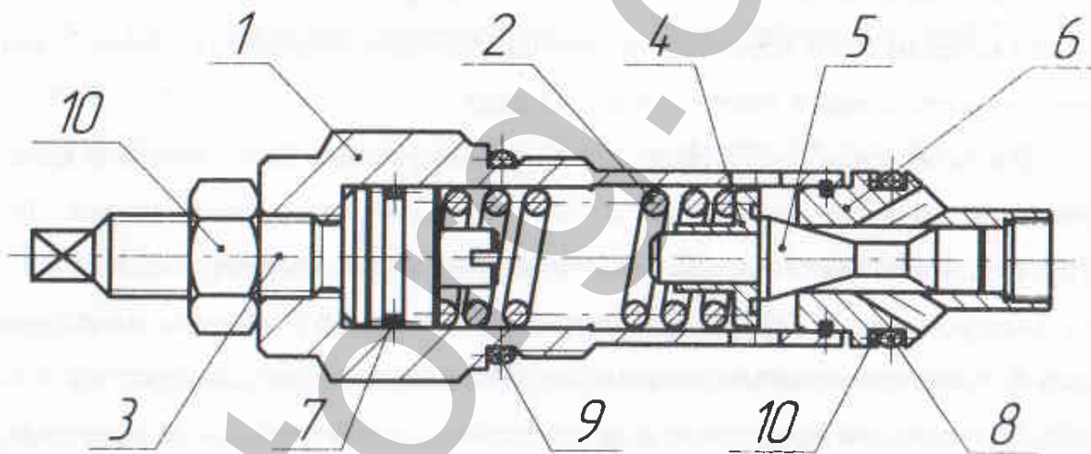
Рисунок 5.2. Клапан предохранительный
