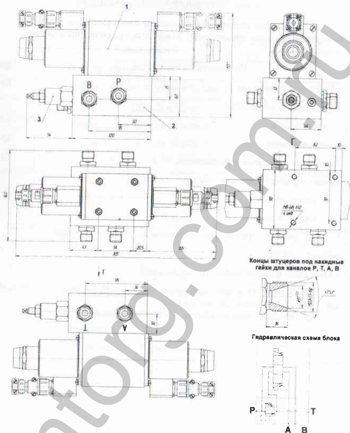
Рис. 1.2. Габаритные и присоединительные размеры блока разгрузки
