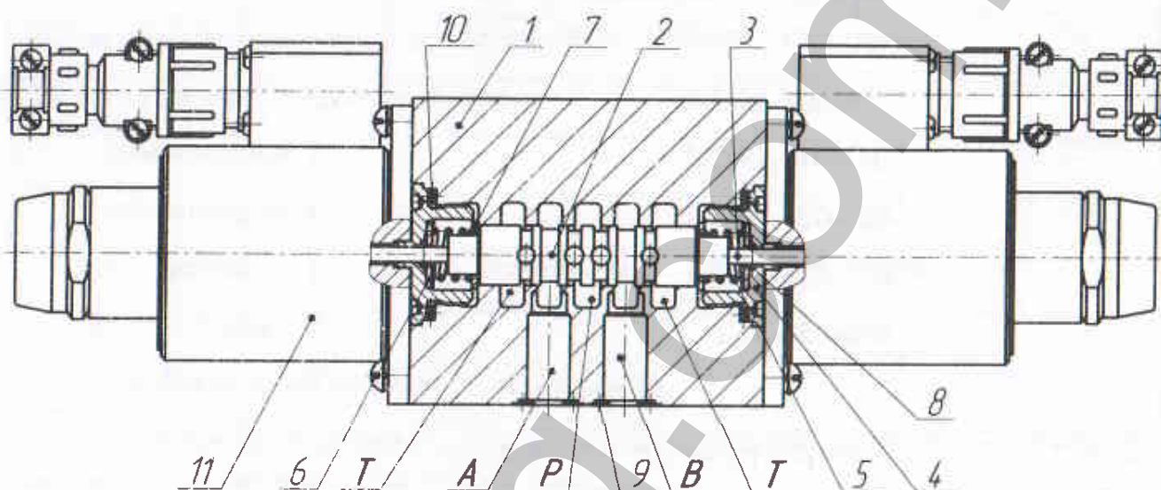
Рисунок 5.1. Конструкция гидрораспределителя
