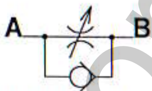
Гидродроссель с обратным клапаном
