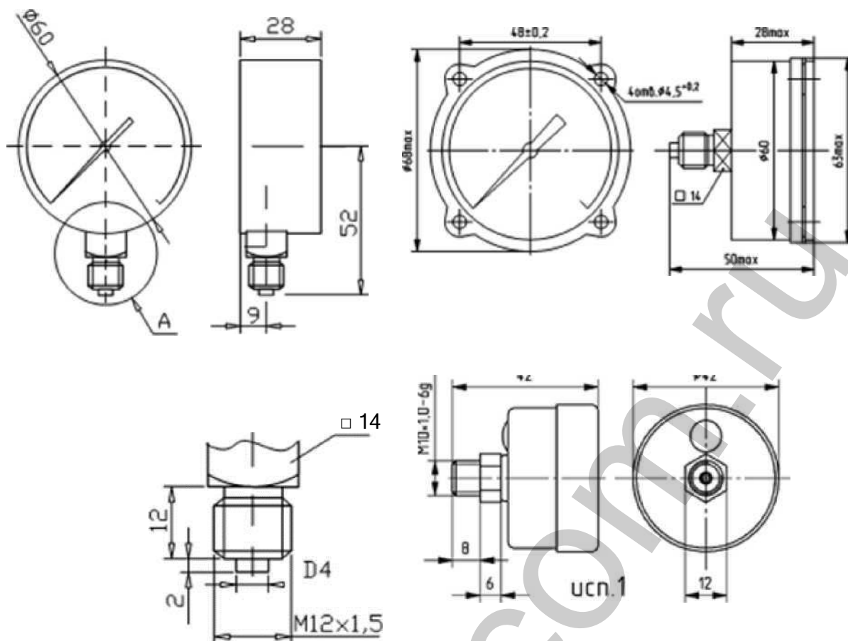
Габаритные и присоединительные размеры МП2-У2
