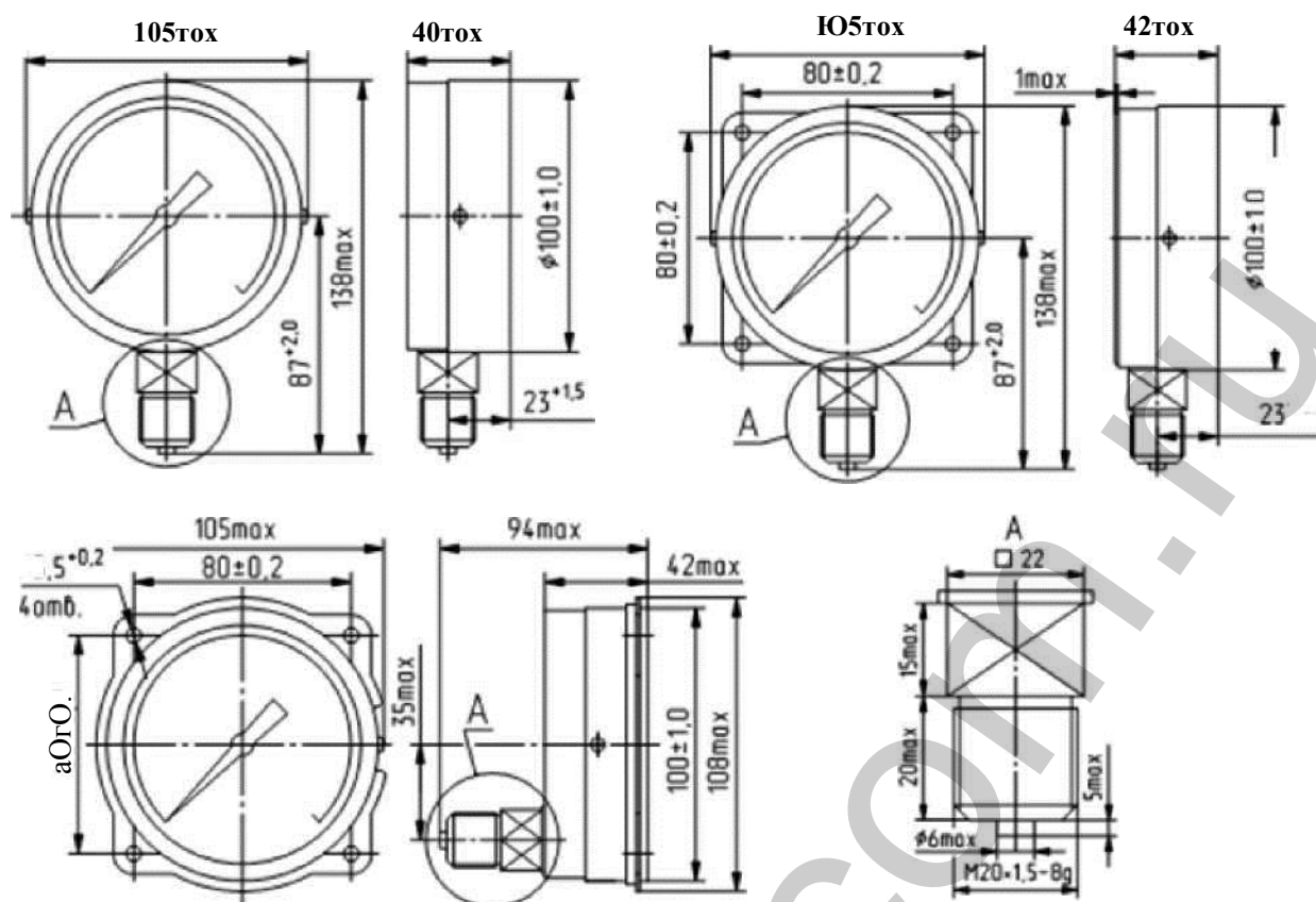
Габаритные и присоединительные размеры МП3А-У2-Кс
