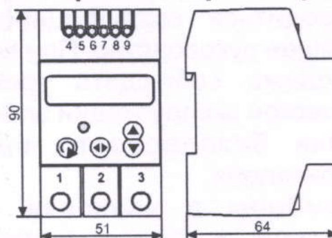
Габаритные размеры
