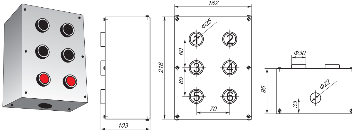
ПК211-6, ПК221-6
