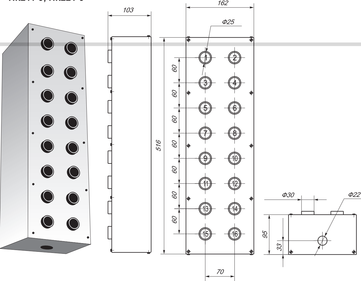
ПК211-9, ПК221-9
