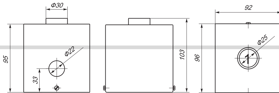
ПК211-1, ПК221-1
