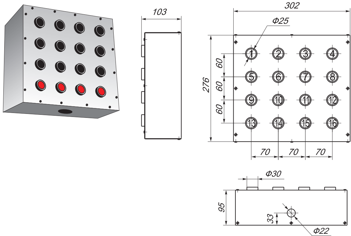
ПК211-9, ПК221-9
