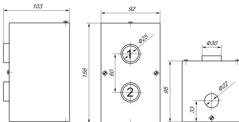
ПК211-2, ПК221-2
