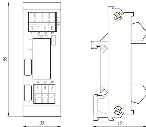
Рисунок 4.1 - Габаритные размеры блока усиления мощности БУМ-1
