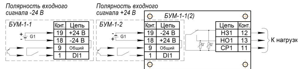
Рисунок 4.2 - Схема подключения БУМ-1
