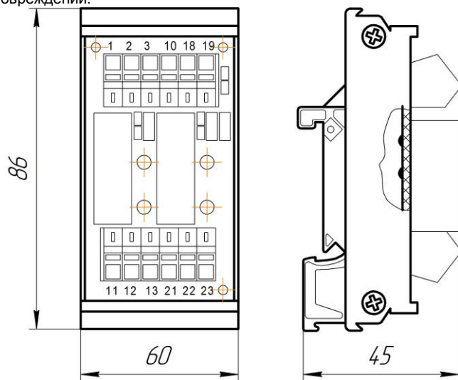
Рисунок 4.1 - Габаритные размеры блока усиления мощности БУМ-2
