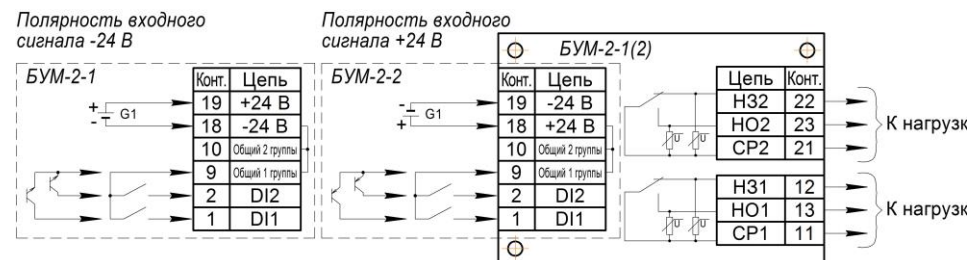
Рисунок 4.2 - Схема подключения БУМ-2
