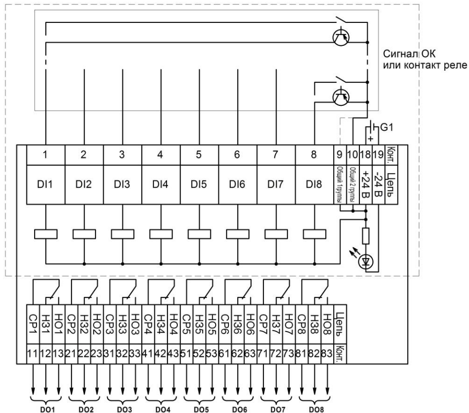
Рисунок 3.2 – Схема внешних соединений БУМ-8Р-1(2)
