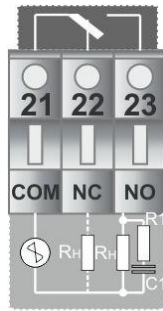
Рисунок Б.2 – Схема подключения индуктивной нагрузки к механическому реле
