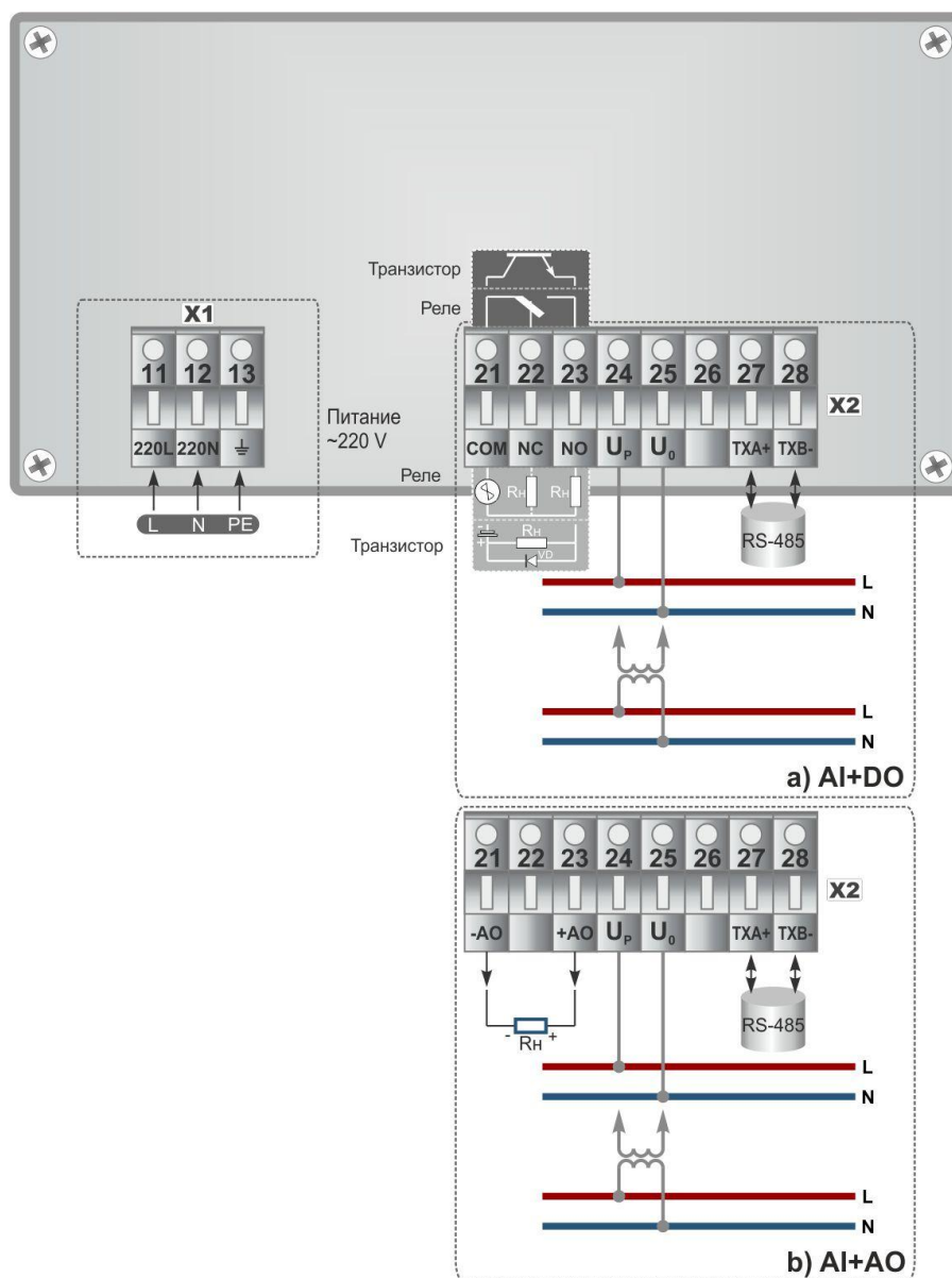
Рисунок Б.1 - Подключение внешних цепей к вольтметру ИПМ-2:
