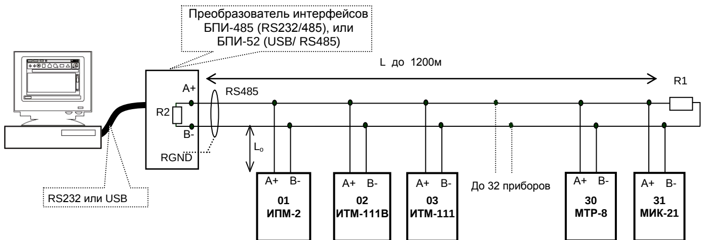
Рисунок Б.3 - Организация интерфейсной связи между компьютером и вольтметрами или контроллерами
