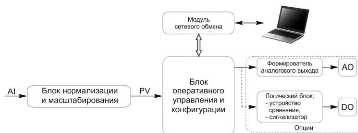
Рисунок 3.3 - Функциональная схема вольтметра ИПМ-2
