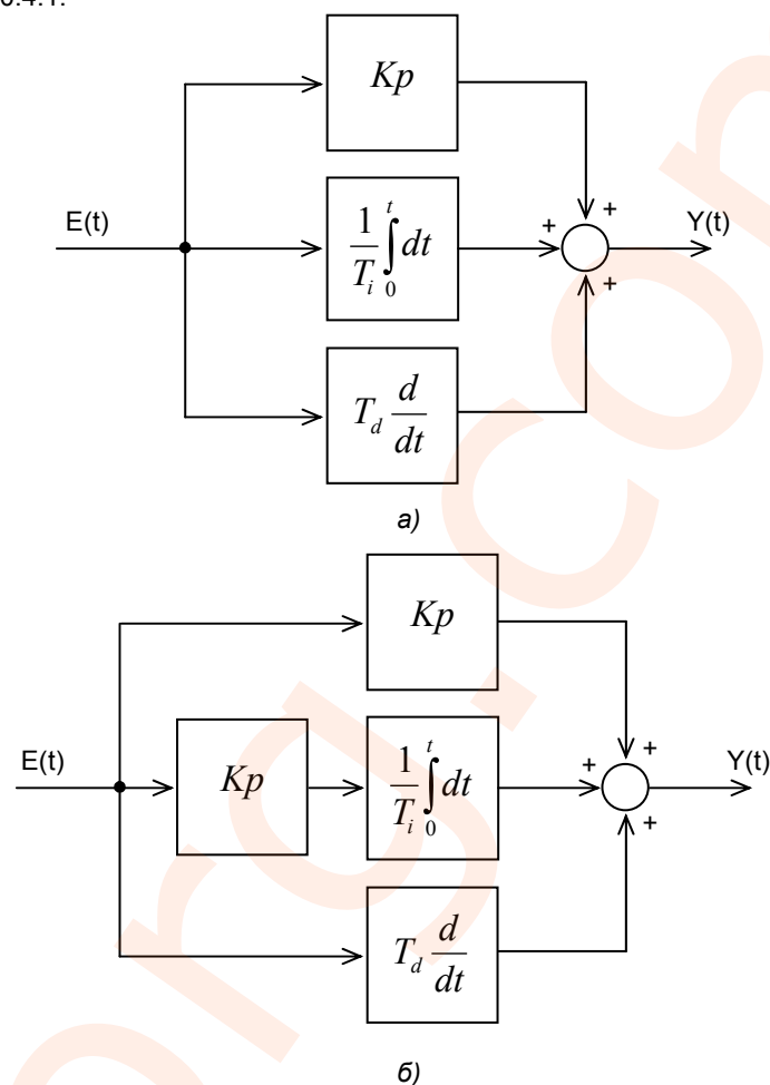
Рисунок 10.4.1. Структуры регуляторов МИК-25:
