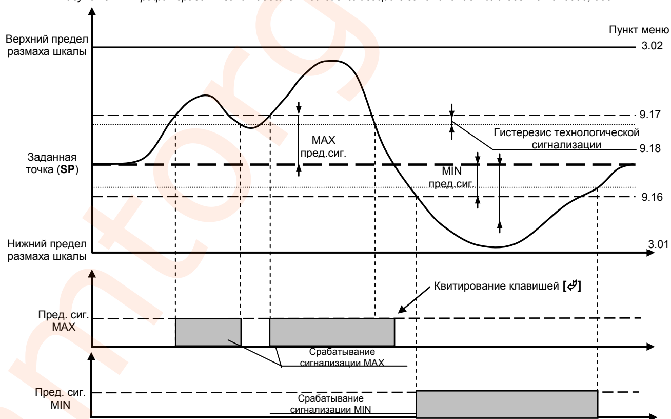
Рисунок 3.13 - График срабатывания девиационной предупредительной сигнализации с запоминанием или без п.9.15=0001, 0003
