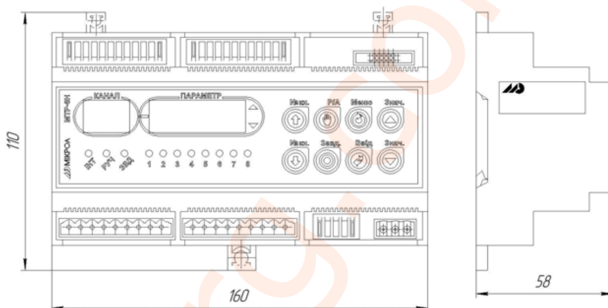
Рисунок А.1 - Габаритные и присоединительные размеры
