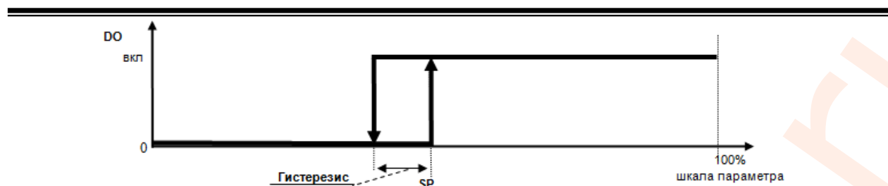
Рисунок 3.10 – Пример работы выходного устройства по логике прямого 2-х позиционного управления п.9.00=0001, п.9.02=0001
