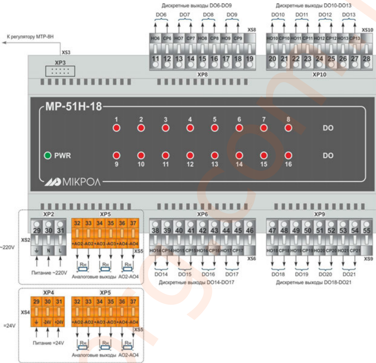
Рисунок Б.11 - Схема внешних подключений модуля расширения МР-51Н-18
