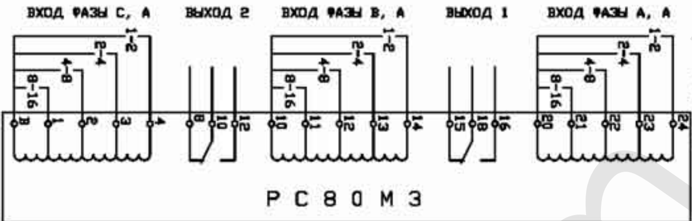
СХЕМА ПОДКЛЮЧЕНИЯ РС80МЗ
