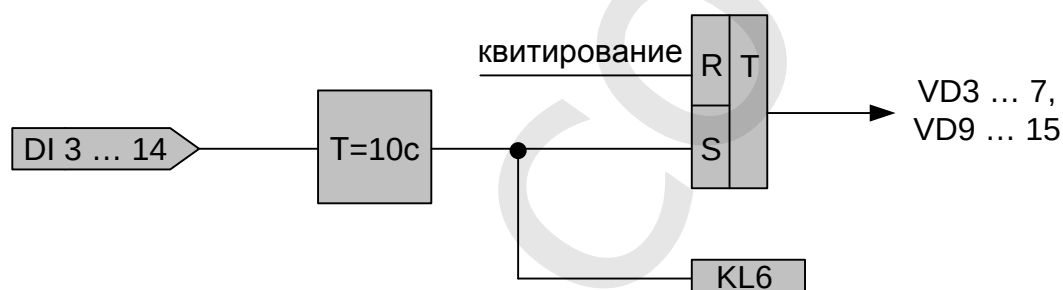
Рис.6. – Блок-схема алгоритма «В»
