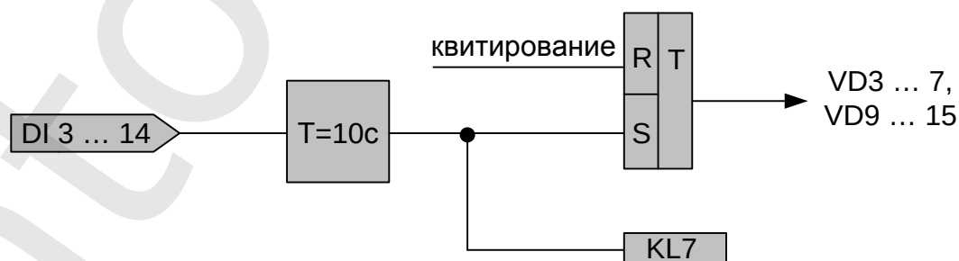
Рис.7. – Блок-схема алгоритма «С»
